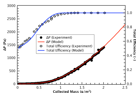
Figure 1. Evolution de la perte de charge et de l'efficacité du filtre E au cours du colmatage – Vitesse de filtration = 2,5 cm/s
