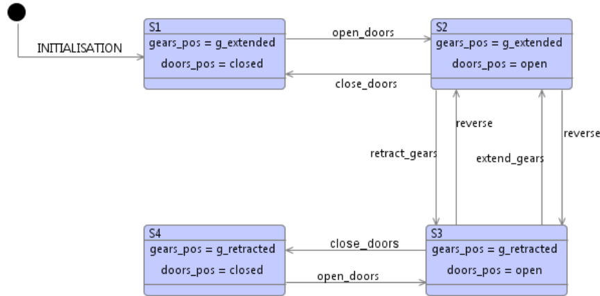
Figure 17: Une sous-machine à états de Landing_System
