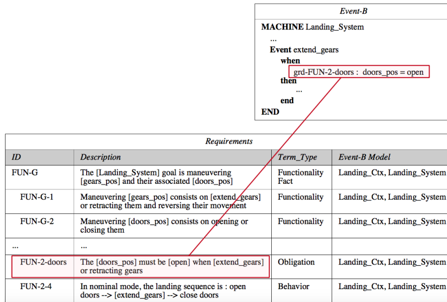
Figure 13: Introduction d'une condition dans un événement existant
