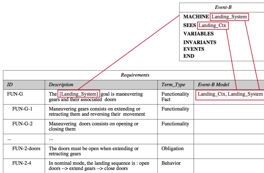
Figure 10: Introduction de la machine et son contexte
