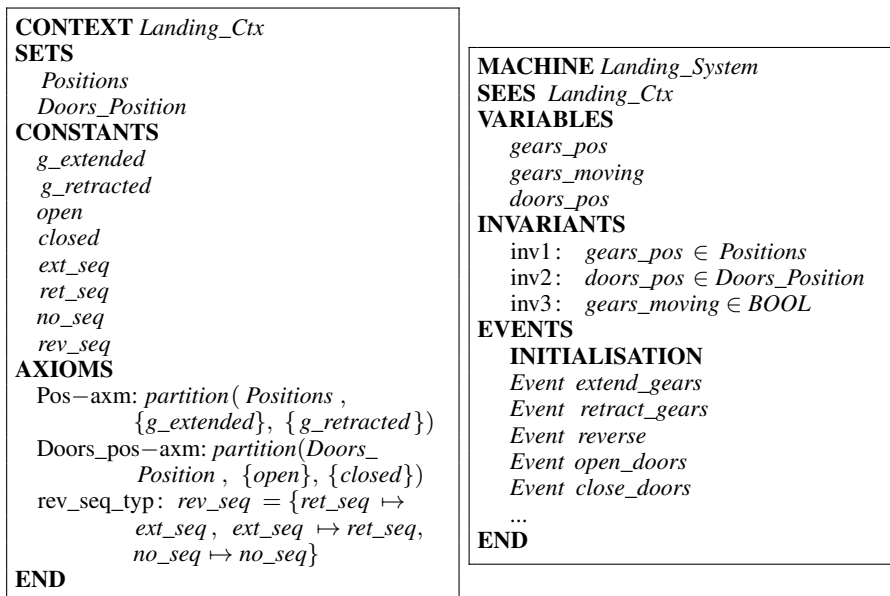
Figure 2: Exemple d'une spécification en Event-B de l'étude de cas choisie
