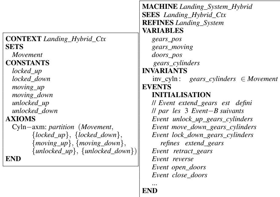
Figure 19: Machine Landing_System_Hybrid et son contexte
