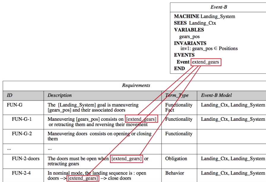
Figure 12: Introduction de la fonctionnalité extend_gears
