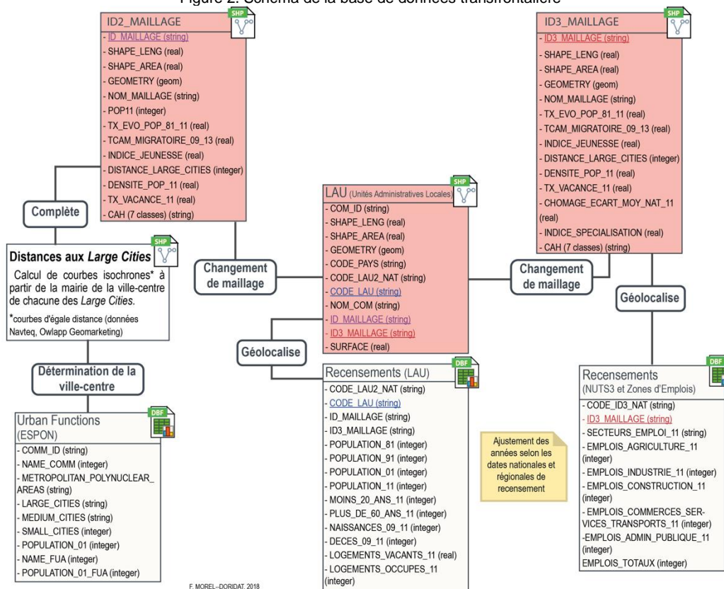
Figure 2. Schéma de la base de données transfrontalière
