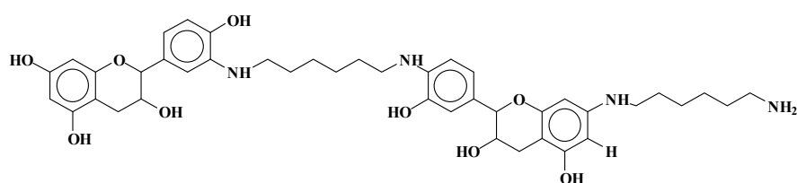
Figure 9. Example of covalent bonds dimer at 758 Da.
