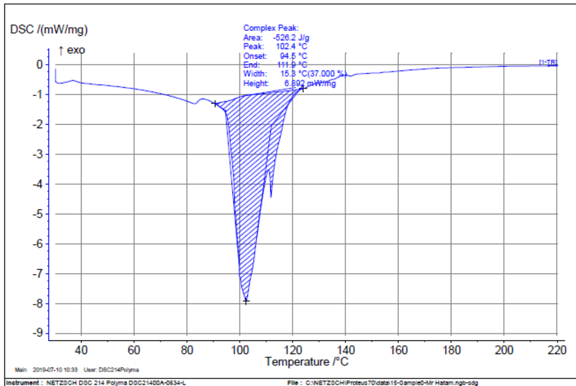
Fig. 1. MF with no TiO 2 . Control
