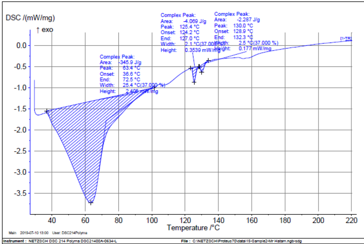
Fig. 3. MF with 2% TiO 2
