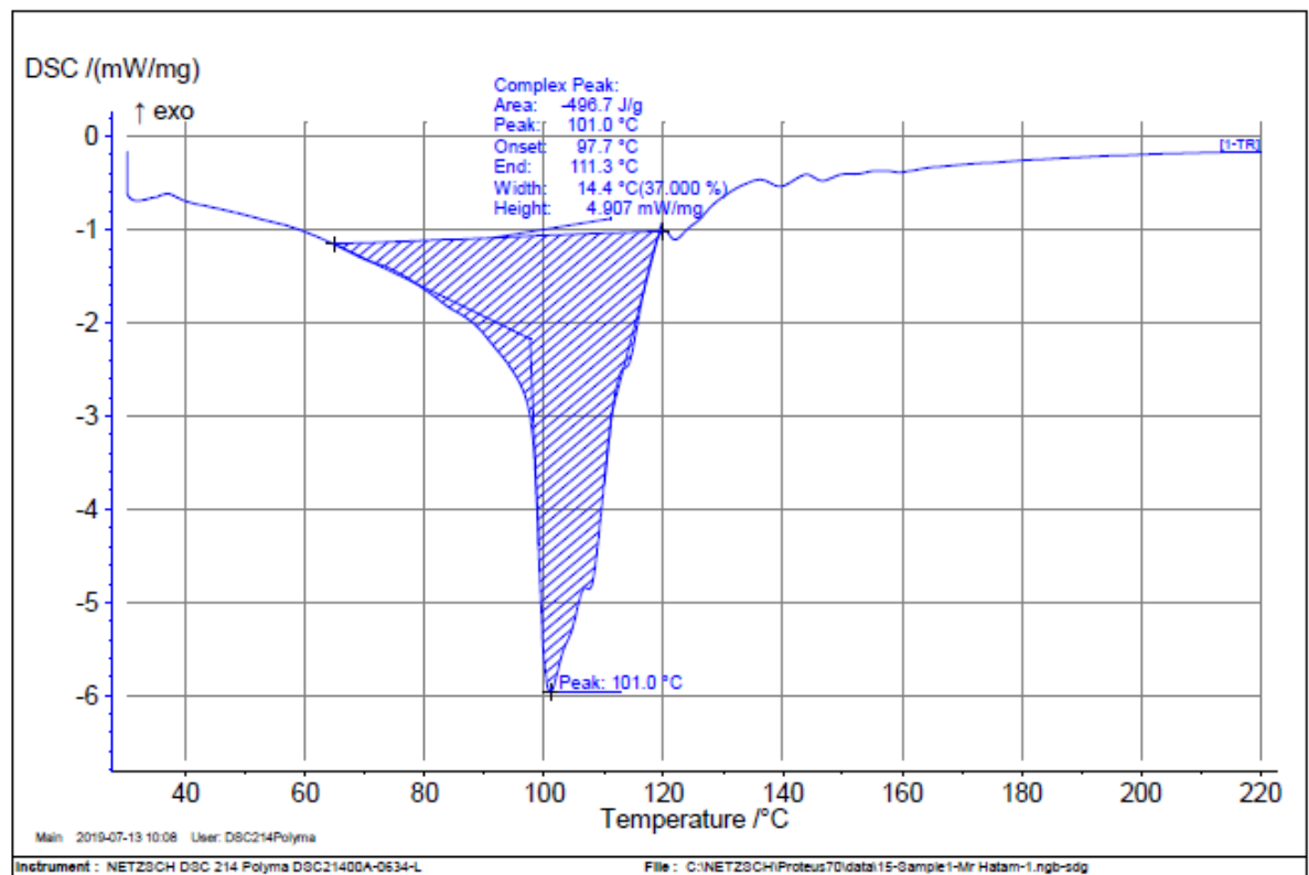
Fig. 2. MF with 1% TiO 2 .
