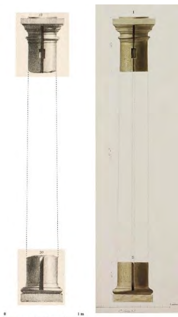
Fig. 4 : Restitution d'une colonne d'ordre dorique de Bleurville (Jollois 1820, feuille n° 5, fig. 1-2, © MDAAC Epinal ; Jollois 1843, pl. 28, fig. 19 et 20)
