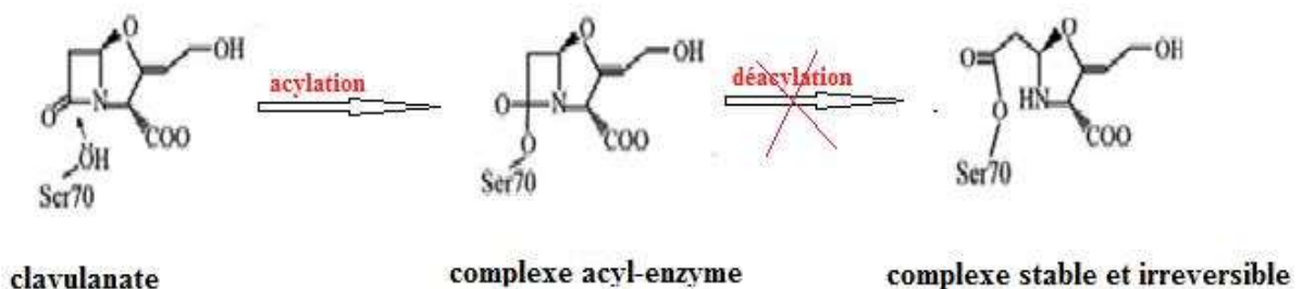
Figure 5 : mode d'action des inhibiteurs des \beta -lactamines (acide clavulanique) (d'après Wright GD, 2000 (23))
