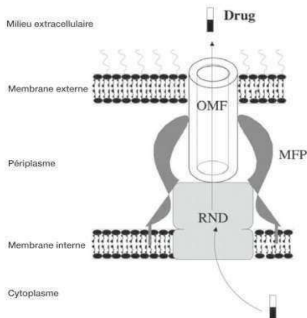
Figure 7 : Système d'efflux tripartite RND d'une bactérie à Gram négatif : RND : Resistance-Nodulation-cell Division, MFP : Membrane Fusion Protein, OMF : Outer Membrane Factor. (d'après Pagès et al., 2011 (28))
