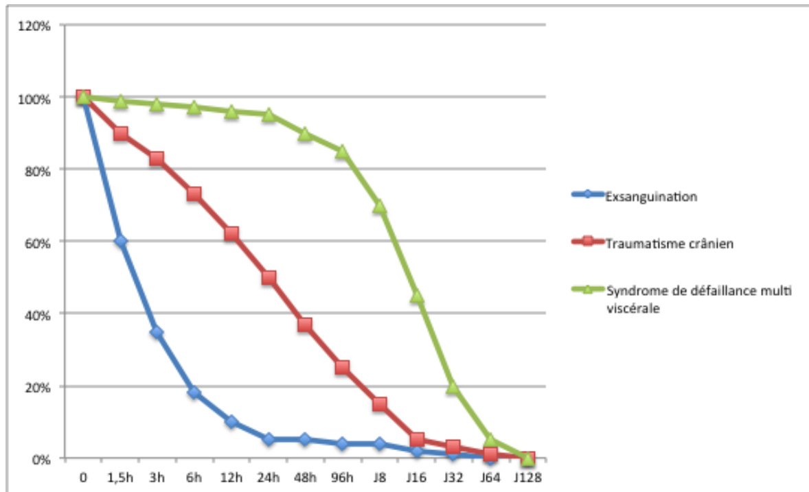
Figure 6: Pourcentage de survie en fonction du temps pour les trois principales causes de décès après un traumatisme selon Dutton et al. (16)
