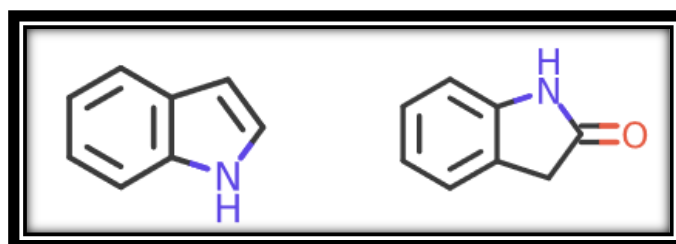
Figure 15: Noyau indole et oxindole
