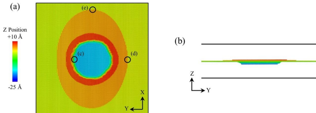
Figure 2 – Simulation par dynamique moléculaire de la formation du cratère après relaxation de la boucle de dislocation dans le joint de macle. (a) Vue de dessus. (b) Vue latérale. En vue de comparer ces résultats à ceux du modèle champ de phase, Y correspond à la direction de maclage, X à la direction transverse et Z à la direction normale.
