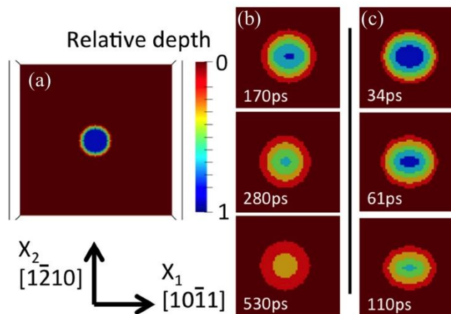
Figure 4 – Simulations de l’annihilation du cratère avec un modèle champ de phase. Les cartes sont coloriées en fonction de la profondeur pour comparer aux simulations de dynamique moléculaire. (a) configuration initiale.
