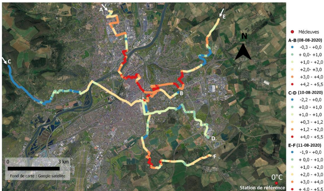
Figure 5 : Ecart de température « instantanés » avec la station rurale de Mécleuves les longs des transects urbains.
