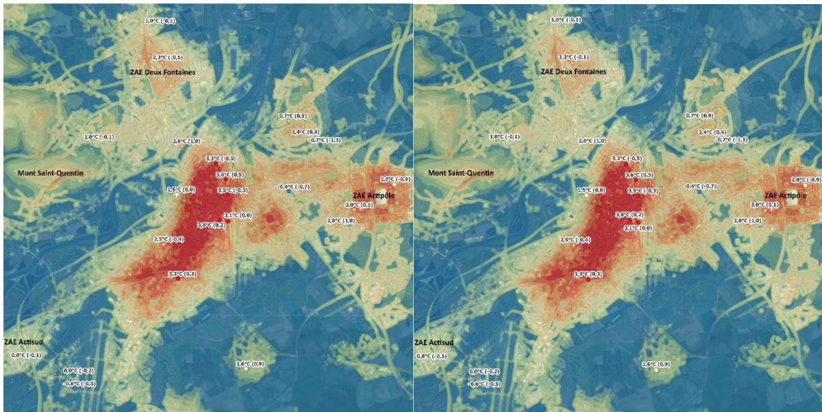
Figure 4 : en haut à gauche, carte de la distribution de l'indice ICU lors de la canicule de juin 2019 (maille 5 x 5 m).
