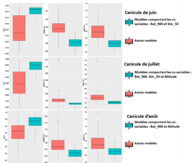
Figure 3 : Boîtes à moustaches représentant les métriques de validation (R 2 , RMSE et MAE) des modèles de régression intégrant (bleues) ou non (rouges) les co-variables les plus fréquentes.
