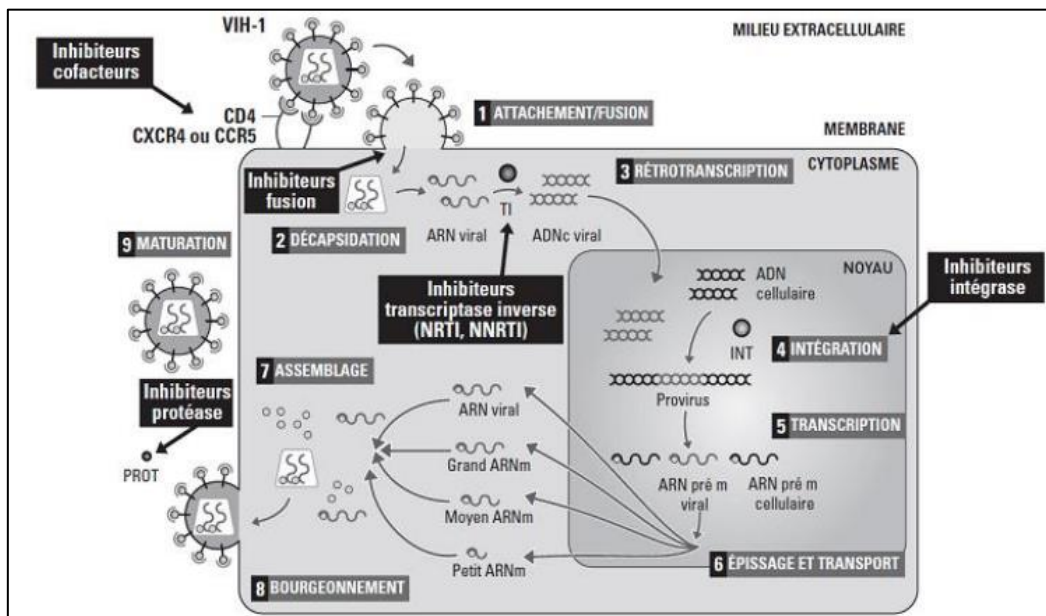
Figure 2. Cycle de réplication du VIH avec sites d'action des principales classes d'antirétroviraux (6)
