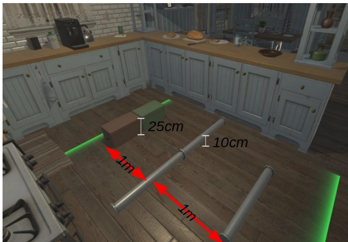
Figure 6. Placement des obstacles sur le parcours
