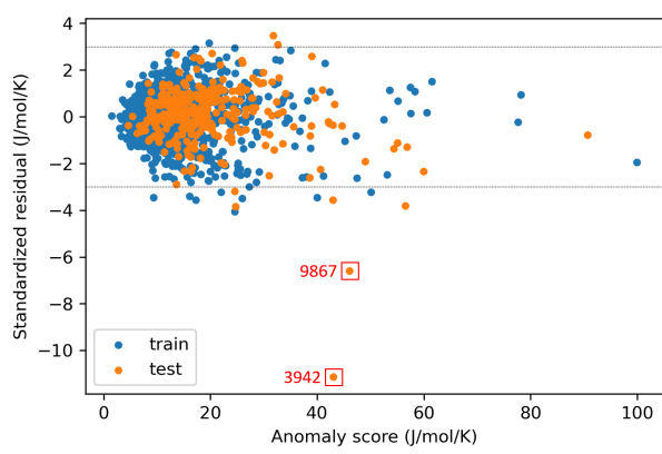
(d) Split 4
