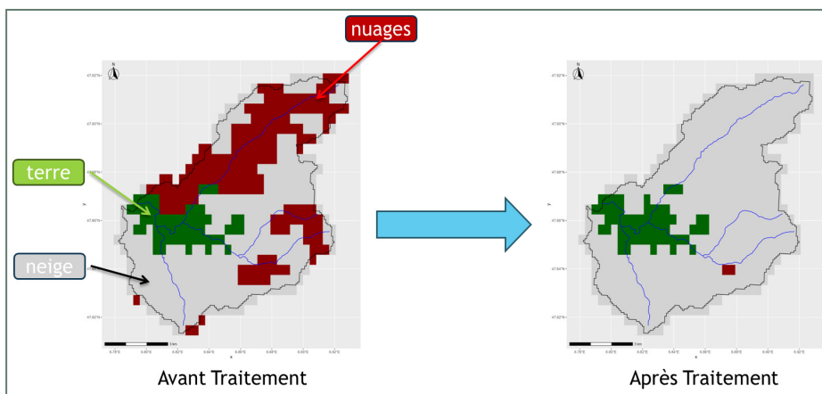
Figure 2 : Exemple d'évolution des images avant et après le traitement (8 janvier 2006)
