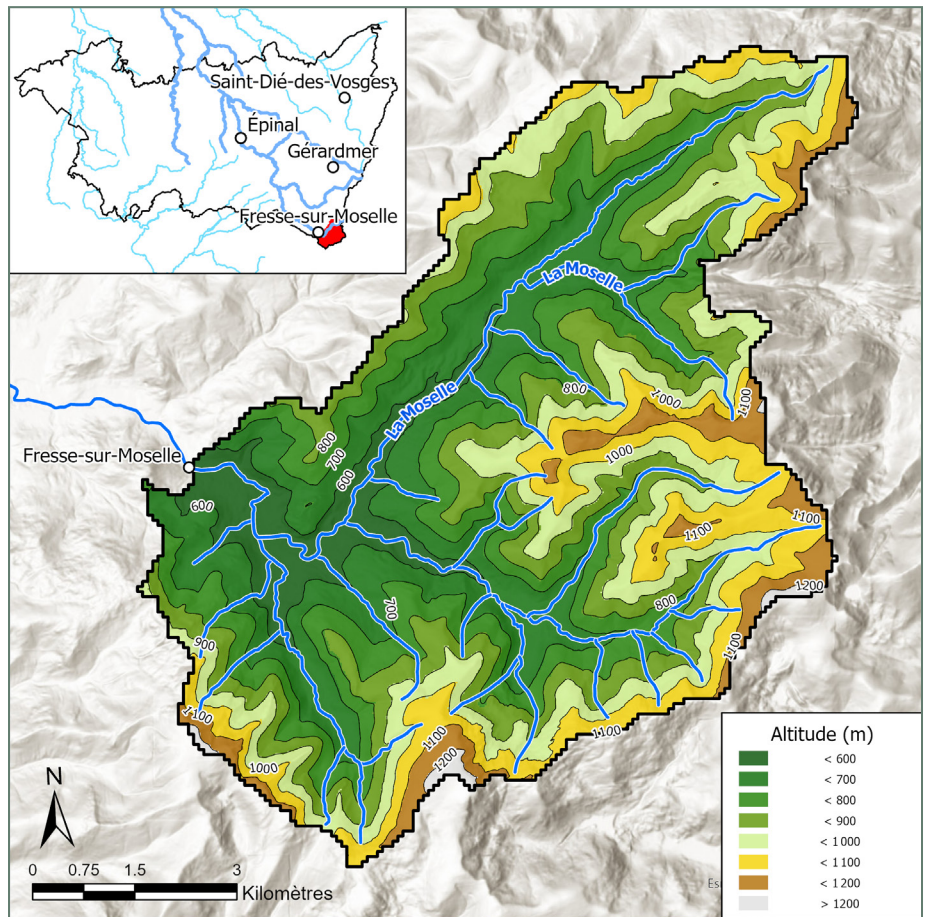
Figure 3 : Localisation et orohydrographie du bassin versant de la Moselle à Fresse-sur-Moselle
