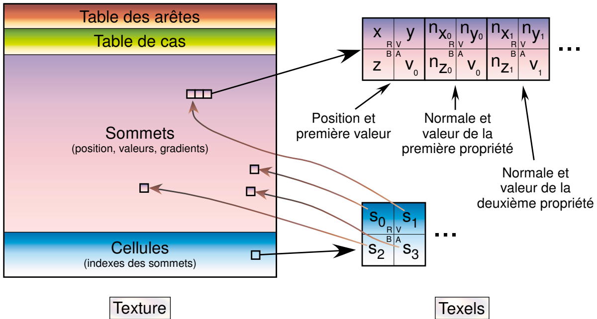
FIG. 1.17 – Stratégie de stockage générique dans une texture des tables d’arêtes et de cas, des sommets (position, valeurs et gradients) et pour chaque cellule, la liste des index (dans la texture) des sommets qui lui sont associés. Plusieurs champs scalaire différents peuvent être attachés à une même grille, c’est pourquoi il est prévu que plusieurs valeurs et gradients puissent être stockés dans la texture pour chaque sommet.
