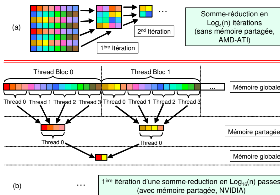
FIG. 2.12 – (a) Parallélisation d’une somme-réduction de vecteur sur une architecture GPU qui ne possède pas de mémoire partagée comme la série X1k d’AMD-ATI. Chaque itération réduit la taille du vecteur d’un facteur 4. (b) La même opération parallélisée sur une architecture GPU qui dispose d’une mémoire partagée comme la série 8 d’NVIDIA. Comme les blocs de threads sont constitués dans cet exemple de quatre threads, chaque itération réduit la taille du vecteur d’un facteur 4 \times 4 = 16 .
