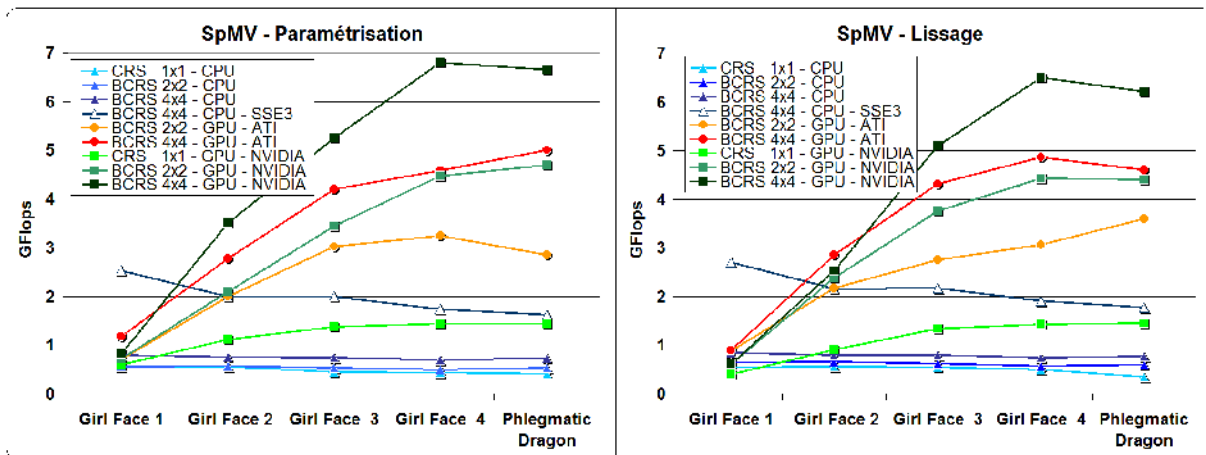
FIG. 2.15 – Comparaison des performances en GFlops de différentes implantations du produit matrice creuse/vecteur (SpMV) dans le cas du calcul d'une paramétrisation de surface et d'un lissage de surface.
