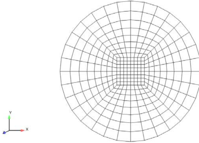
FIGURE 3.3 – Section transversale du maillage de la conduite pour l'expérience de Liu et Agarwal [38]
