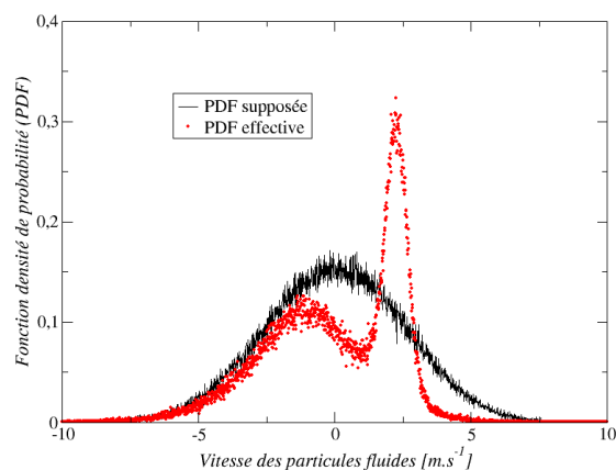
FIGURE 6.6 – Différence entre la PDF des vitesses supposée (points noirs) et effective (points rouges)
