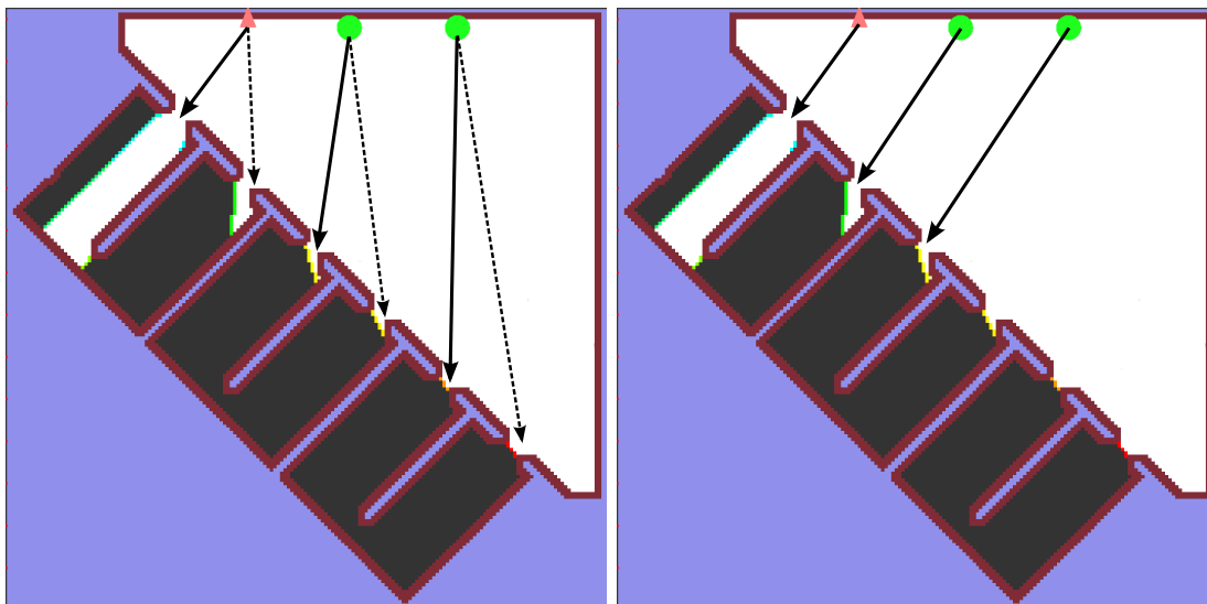
FIGURE 4.9 – Affectation de MinPos (à gauche) et l'affectation gloutonne (à droite) sur l'environnement écurie. Les flèches (en ligne pleine) illustrent l'affectation, celles en pointillé montrent les deuxièmes frontières pour lesquelles les robots sont en première position.
