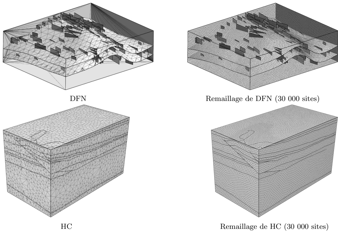
FIGURE 4.13 – REMAILLAGE DES MODÈLES DFN ET HC. (voir les tableaux 4.1 et 4.2 pour des détails).
