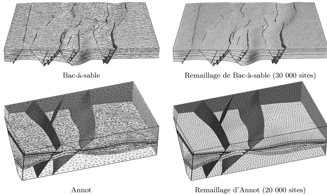
FIGURE 4.18 – REMAILLAGE DE MODÈLES PARTICULIÈREMENT COMPLICQUÉS : BAC-À-SABLE ET ANNOT. (voir les tableaux 4.1 et 4.2 pour des détails)
