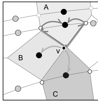
FIGURE 5.5 – DÉTERMINATION DES SOMMETS D'UNE CELLULE DUALE D'UN SOMMET DU DIAGRAMME DE VORONOÏ.
