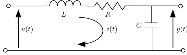
FIGURE 1.8 – Circuit électrique RLC.
