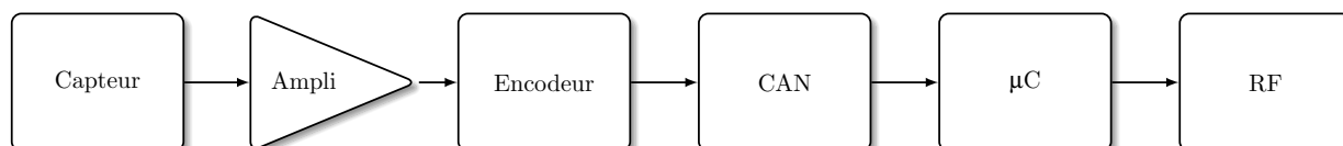
FIGURE 4.3 – Modèle d'un nœud avec encodeur AC.
