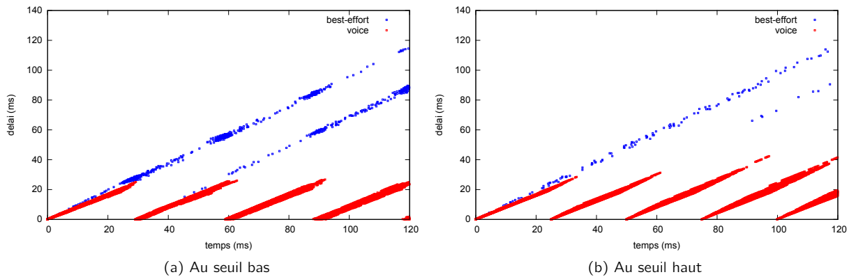
Figure 3.60 – Évolution du délai lorsque le flux best-effort est agrégé ( e500v_{e50} )
