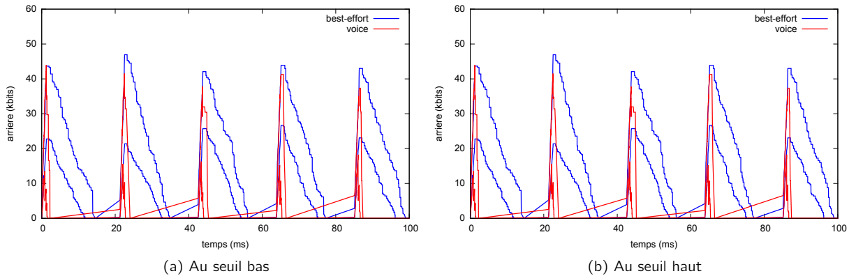
Figure 3.37 – Évolution de l'arrière de traitement lorsque le flux voice est agrégé ( e_{125}v_{e40} )
