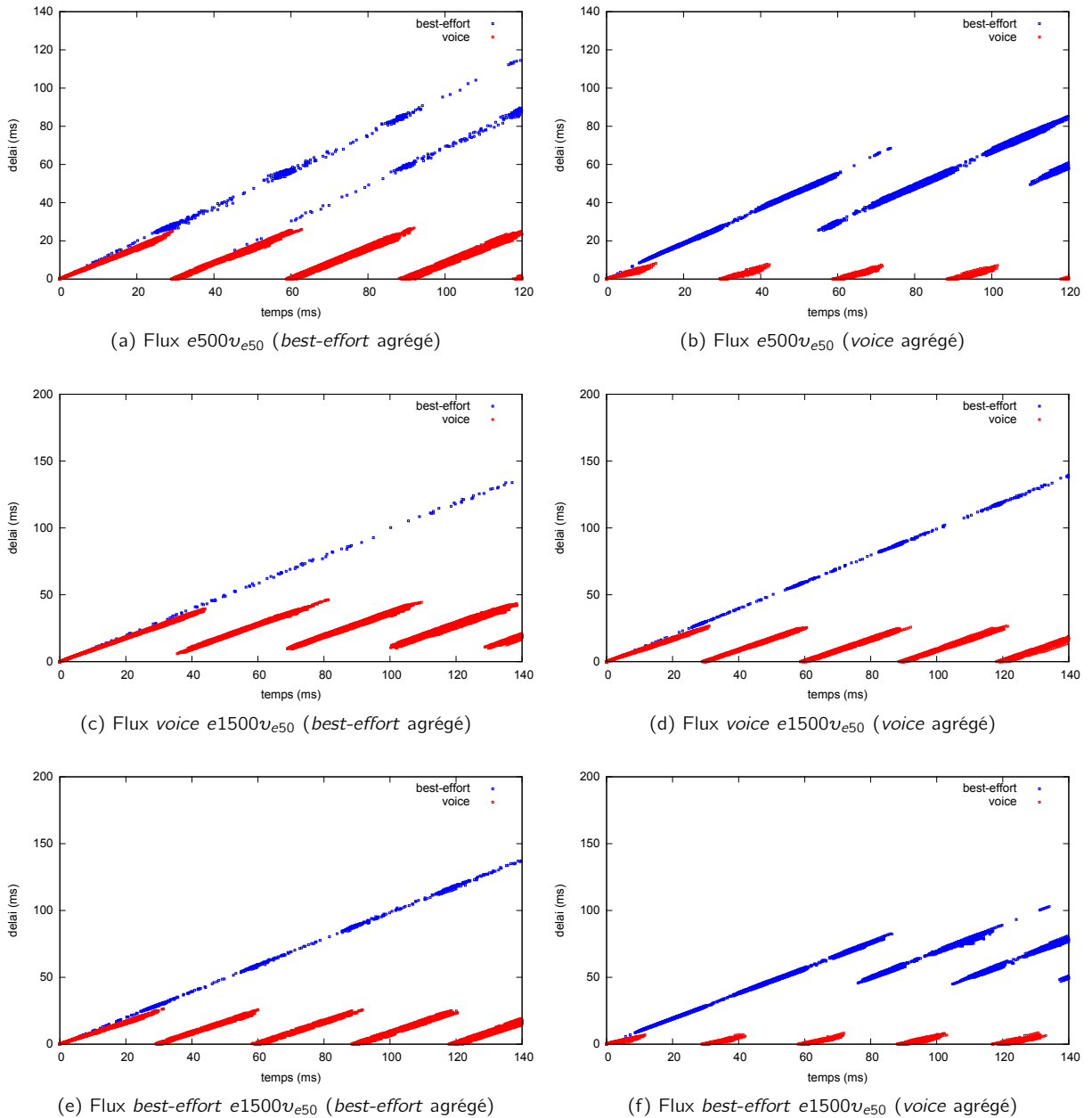
Figure 3.30 – Évolution du délai lors de l'augmentation de taille des paquets (un seul flux agrégé)
