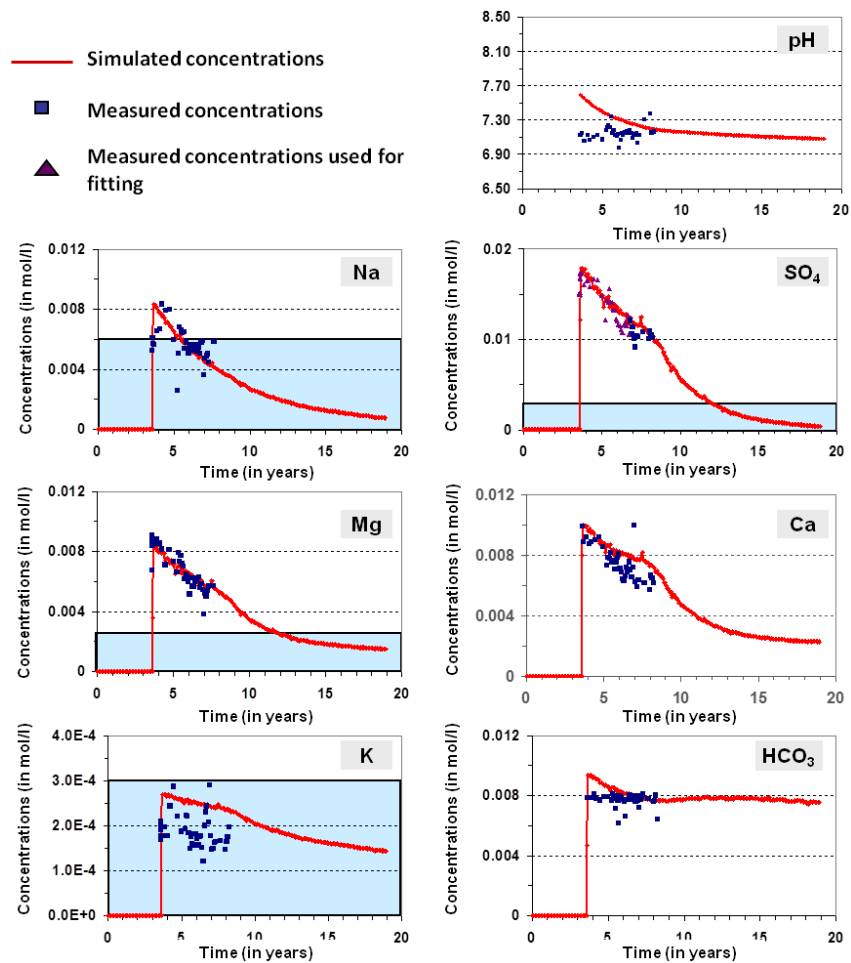
Figure II.5 : Concentrations mesurées et concentrations simulées par le modèle de réacteurs en réseaux au point de débordement du bassin sud du BFL (modifié d'après Collon et al. (2006)). La zone bleu correspond à la concentration maximale autorisée pour l'alimentation en eau potable. Elle n'est pas indiquée pour le Ca et le HCO_3 car dans ces deux cas la norme est toujours respectée.
