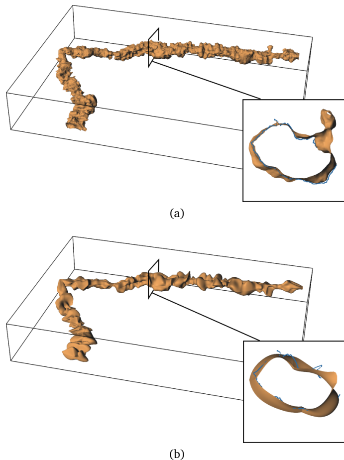
Figure II.41 : Résultats de la reconstruction 3D du conduit karstique exploré par laser optique présenté en figure II.40 (modifié d'après Lavandier et al. (2015)) : (a) réalisation obtenue avec la méthode ODSIM utilisant l'échantillonneur de Gibbs et la complétion automatique de données ; (b) réalisation avec l'approche basée sur l'interpolation itérative de surface paramétrique.
