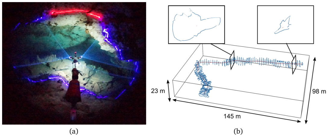
Figure II.40 : Système d'acquisition par laser optique : (a) exemple de mise en œuvre du dispositif pour l'acquisition d'une section ; (b) ensemble de données résultant de l'exploration d'un tunnel (85 sections) (Schiller and Renard, 2016).
