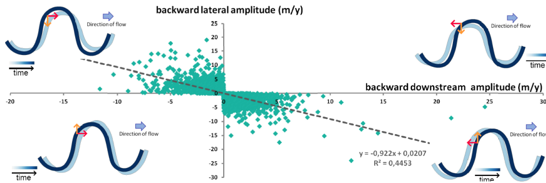
Figure II.36 : Amplitudes de migration latérale vs. amplitudes de migration avale mesurées sur 4 lits successifs du fleuve Mississippi (données publiques de l'armée américaine 1 ) : une anti-corrélation est observée (Parquer et al., 2016a).
