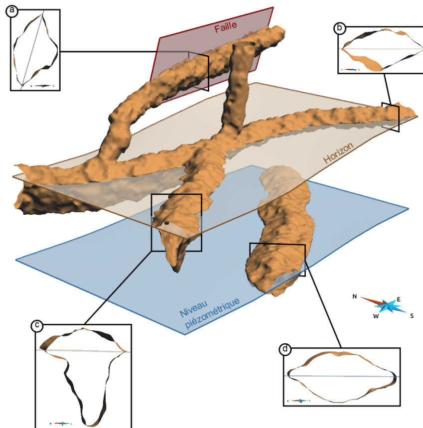
Figure II.39 : Conduit simulé à partir d'un plan d'inception stratigraphique (horizon), d'un plan d'inception tectonique (faille) et d'un niveau d'attraction superposé au niveau piézométrique. Tous ces éléments sont pris en compte dans la morphologie des conduits simulés (Rongier and Collon, 2014).
