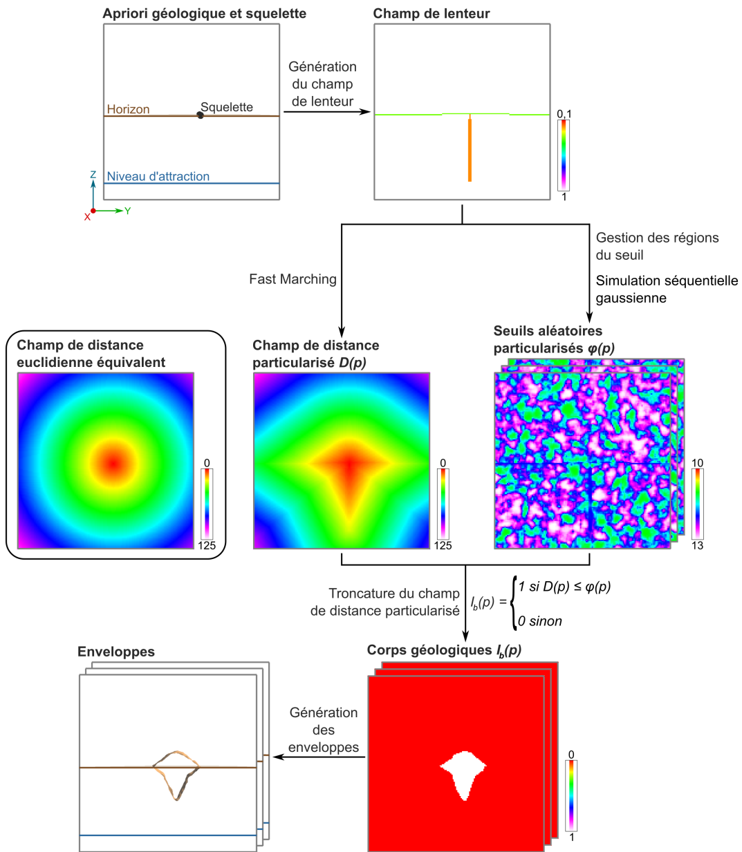
Figure II.38 : Étapes de génération des enveloppes produisant plusieurs représentations possibles d'un conduit karstique (Rongier and Collon, 2014). Le champ de lenteur correspond à l'inverse du champ de vitesse. Le champ de propagation affiche clairement la forme en trou de serrure du conduit, là où le champ de distance euclidienne affiche une forme purement circulaire. Les étapes sont présentées à l'aide de sections 2D pour plus de clarté mais les enveloppes sont générées directement en 3D.
