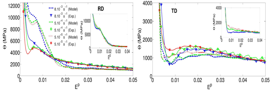
FIGURE 3.12 – Comparaisons des évolutions des taux d'écroûissage entre expériences et simulations. En encart : résultats des simulations avec les mêmes valeurs de n et C_1 sur toutes les familles de glissement ( n = 50 et C_1 = 1.5 \cdot 10^{-4} ).
