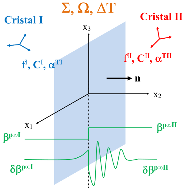
FIGURE 2.3 – Bicristal infini avec interface plane et variations possibles des distorsions plastiques le long de la normale à l'interface.
