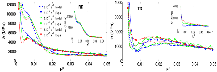
FIGURE 3.12 – Comparaisons des évolutions des taux d'écoulement entre expériences et simulations. En encart : résultats des simulations avec les mêmes valeurs de n et C_1 sur toutes les familles de glissement ( n = 50 et C_1 = 1.5 \cdot 10^{-4} ).
