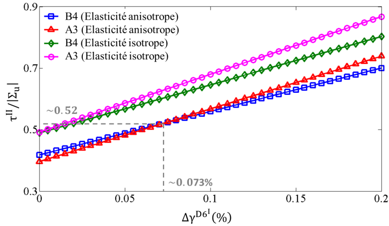
FIGURE 2.7 – Variation des cisssions résolues sur les systèmes A3 et B4 dans le cristal II en fonction de l'amplitude du glissement sur le système D6 dans le cristal I \Delta\gamma^{D6^I} . Comparaison entre les prédictions des formulations anisotrope et isotrope.
