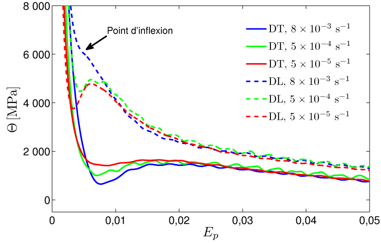
FIGURE 3.11 – Evolution du taux d'érouissage en fonction de la déformation plastique.
