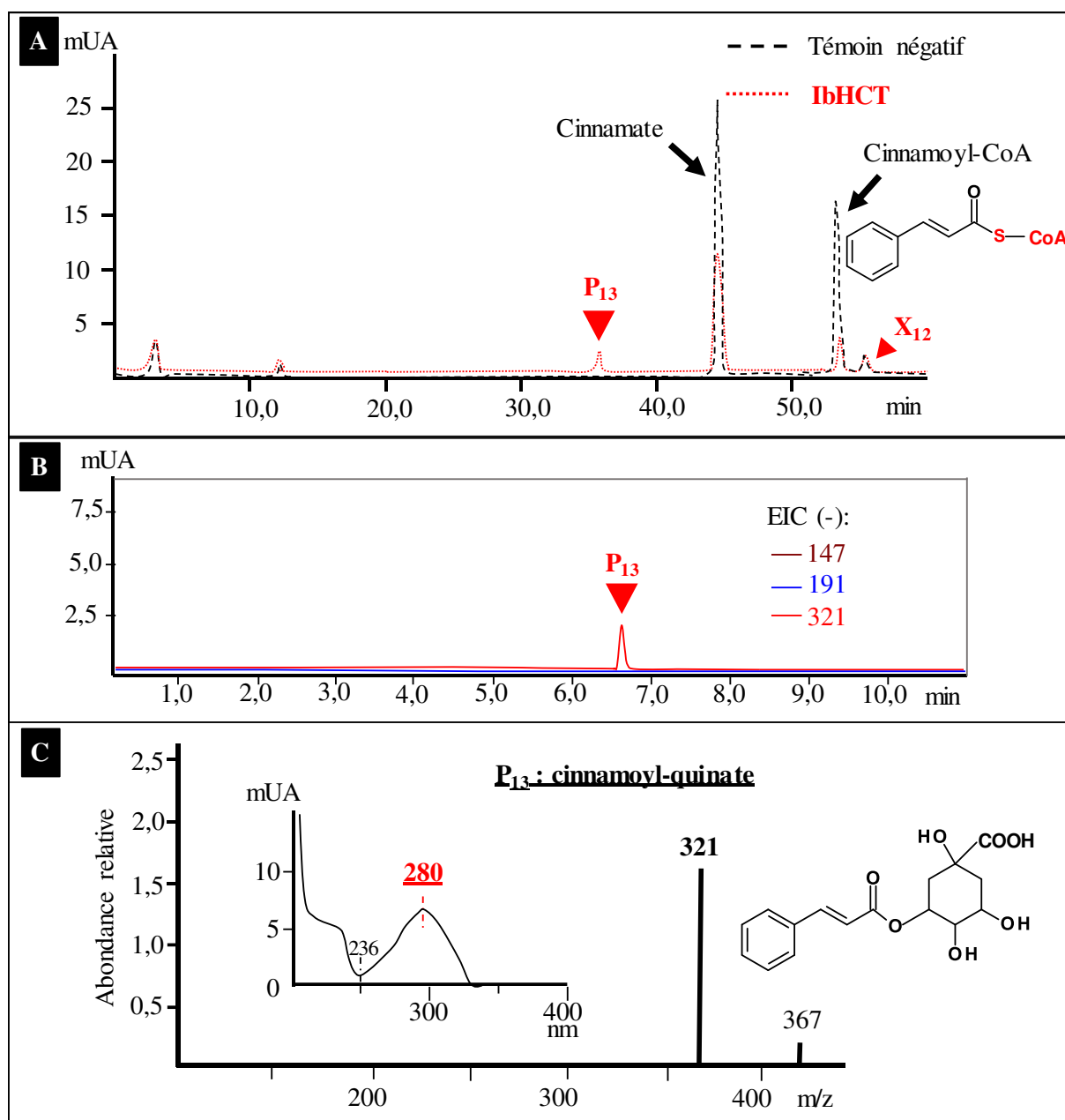
Figure 64 : Synthèse de cinnamoyl-quinate par l'HCT d'ipomée à partir de cinnamoyl-CoA et de quinate. A : chromatogramme HPLC à 310nm. B : chromatogramme MS en mode négatif
