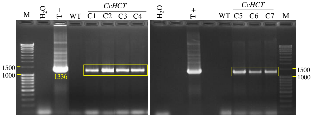
Figure 70 : Sélection des plantes transformées par PCR. Amplification du gène CcHCT (1336 pb). WT : plante sauvage (non transformée).
