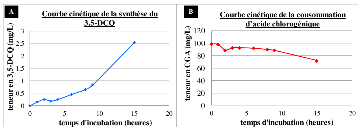
Figure 54 : Étude cinétique de la formation de 3,5-DCQ (A) et de la consommation d'acide chlorogénique en fonction du temps (B).
