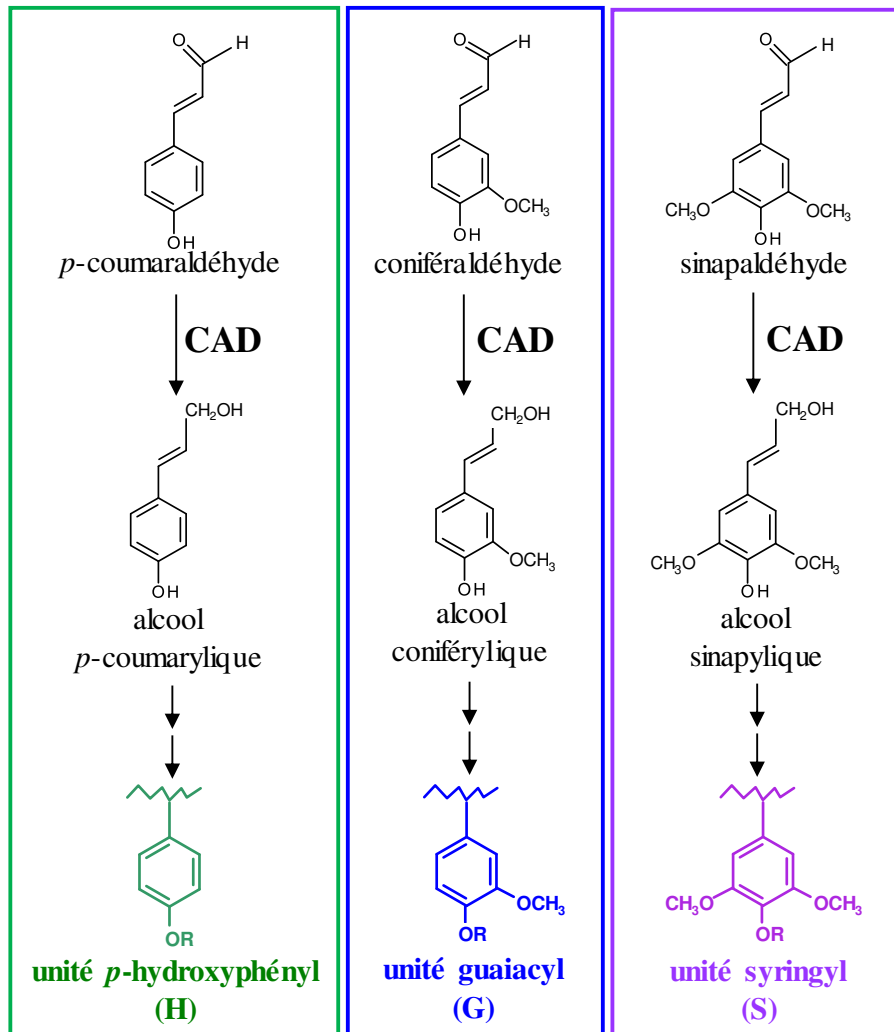
Figure 8 : Structure et formation des trois unités monolignols composant les lignines. CAD : cinnamyl alcohol deshydrogenase.
