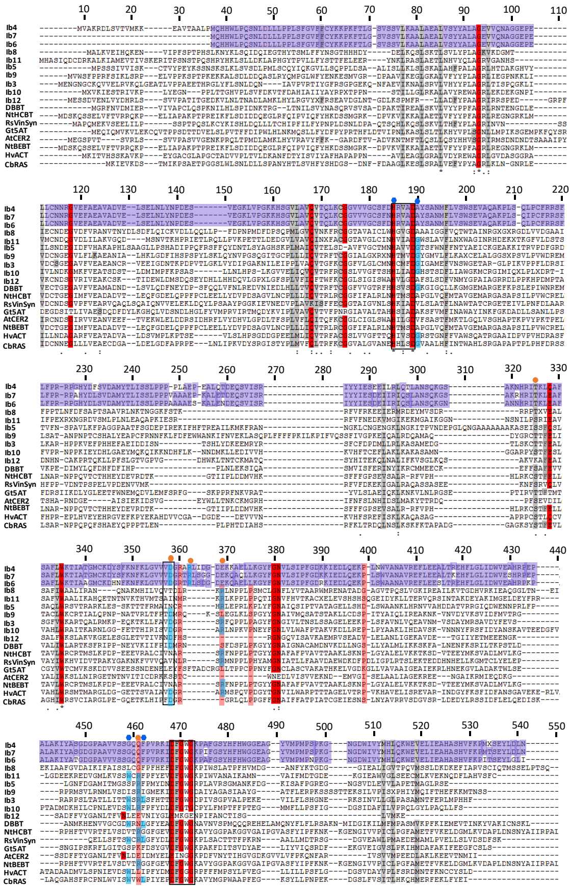
Figure 32 : Alignement des séquences candidates Ib3 et Ib12 avec des membres représentatifs de la famille des BAHD. Les résidus conservés à 95% sont surlignés en rouge et
