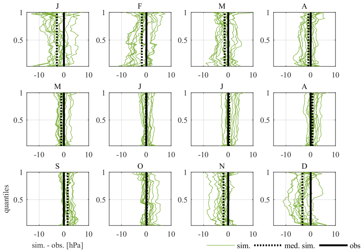
FIGURE 3.3 – Courbes des écarts entre les fréquences cumulées des données de P_{\text{mer}} simulées par les MCGs (cf. Tableau 3.1) et des données observées, période 1979-2005, point de grille 5^{\circ}\text{E}-50^{\circ}\text{N} .
