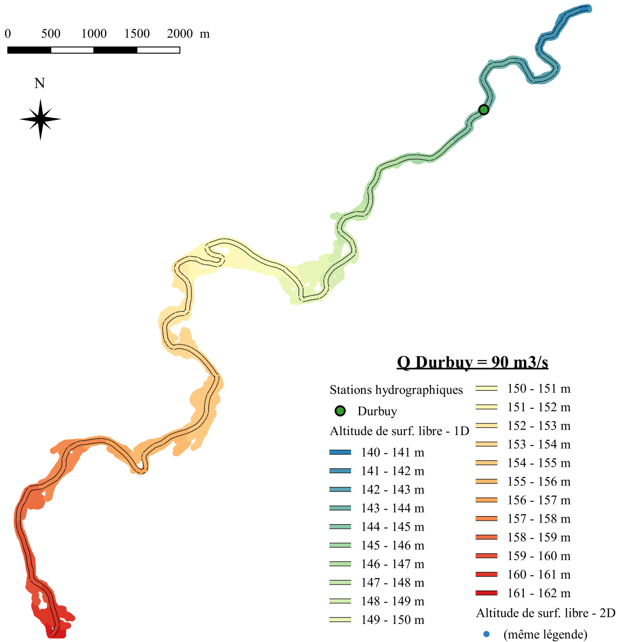
FIGURE 7.7 – Comparaison de l’altitude de surface libre indiquée par le modèle 2D (aplats de couleur) et par le modèle 1D (encadré par les deux traits noirs), pour un débit à Durbuy de 90 \text{ m}^3/\text{s} . L’échelle de couleur pour la représentation des altitudes est identiques pour les deux simulations. Tronçon de l’amont à l’aval de Durbuy.
