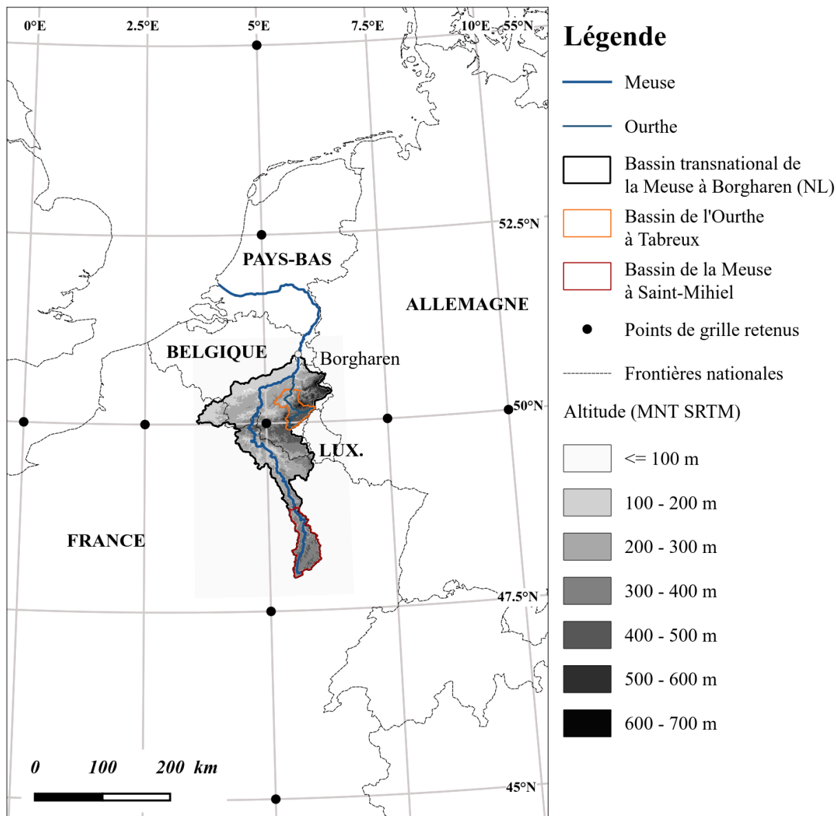
FIGURE 4.1 – Limites des bassins versants étudiés et positionnement des points de grille utilisés pour le calcul de l'indice atmosphérique « pression gradient force » (PGF) de Kastendeuch (2007)
