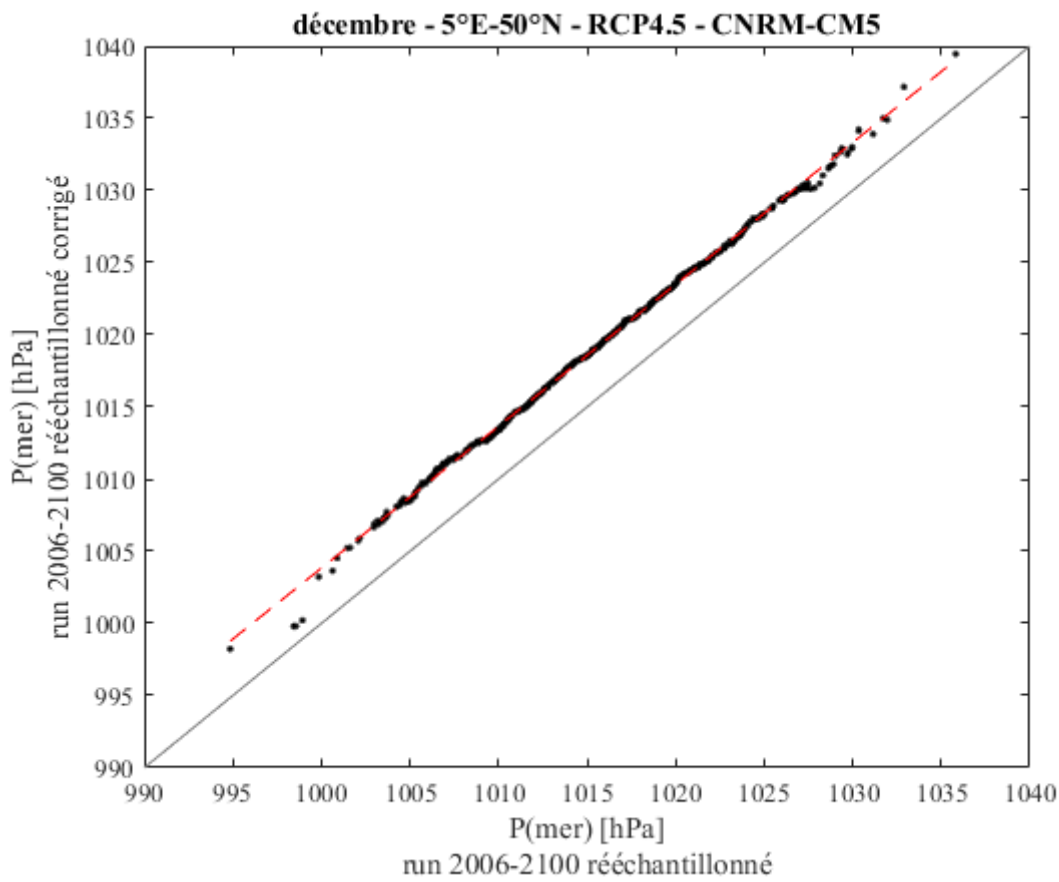
FIGURE 3.10 – Nuage de corrélation et droite de régression utilisée pour débiaiser les données mensuelles brutes de P_{\text{mer}} issues du run forcé RCP 4.5 du modèle CNRM-CM5 (point de grille 5°E-50°N). Les résultats concernent le mois de décembre.
