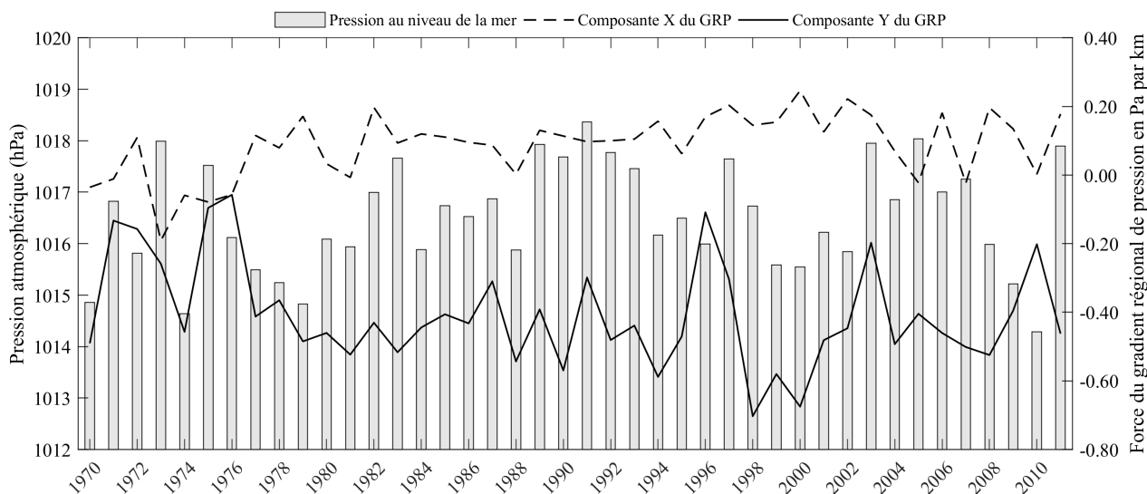
FIGURE 4.3 – Chronique annuelle des composantes X_{PGF} et Y_{PGF} du « pressure gradient force » (PGF) et de la pression atmosphérique au niveau de la mer au point de grille 5^{\circ}E , 50^{\circ}N sur la période 1970-2011. X_{PGF} et Y_{PGF} ont été calculés à partir de la pression au niveau de la mer et d’une grille de 2.5^{\circ} de résolution.
