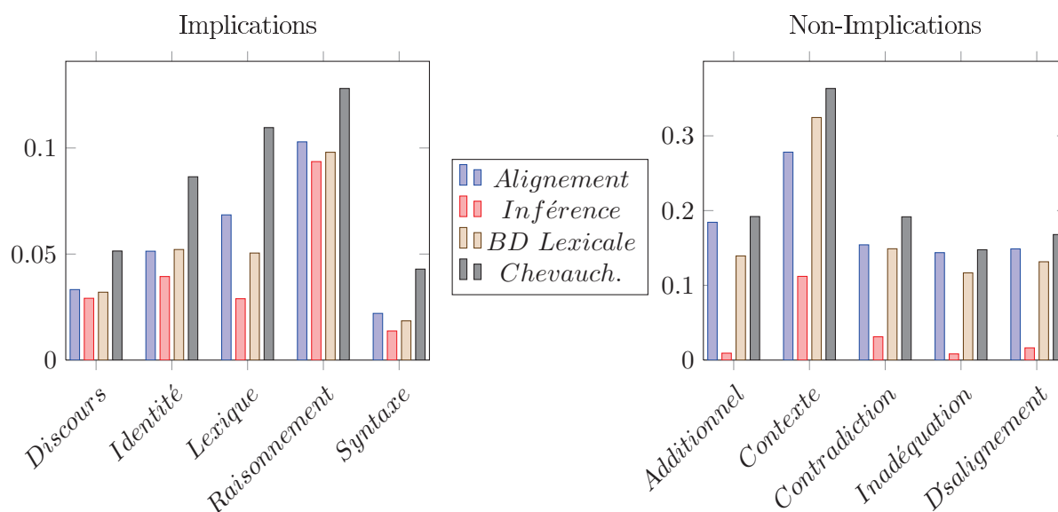
FIGURE 5.3 – Résultats de la fouille d’erreurs appliqué à l’ensemble des couples (type de système, phénomène). L’ordonnée représente la suspicions pour chaque couple (type de système, phénomène).
