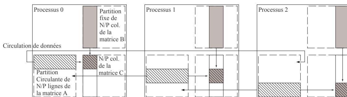
FIGURE 5.5 – Produit de matrice denses en parallèle sur un anneau de processeurs.
