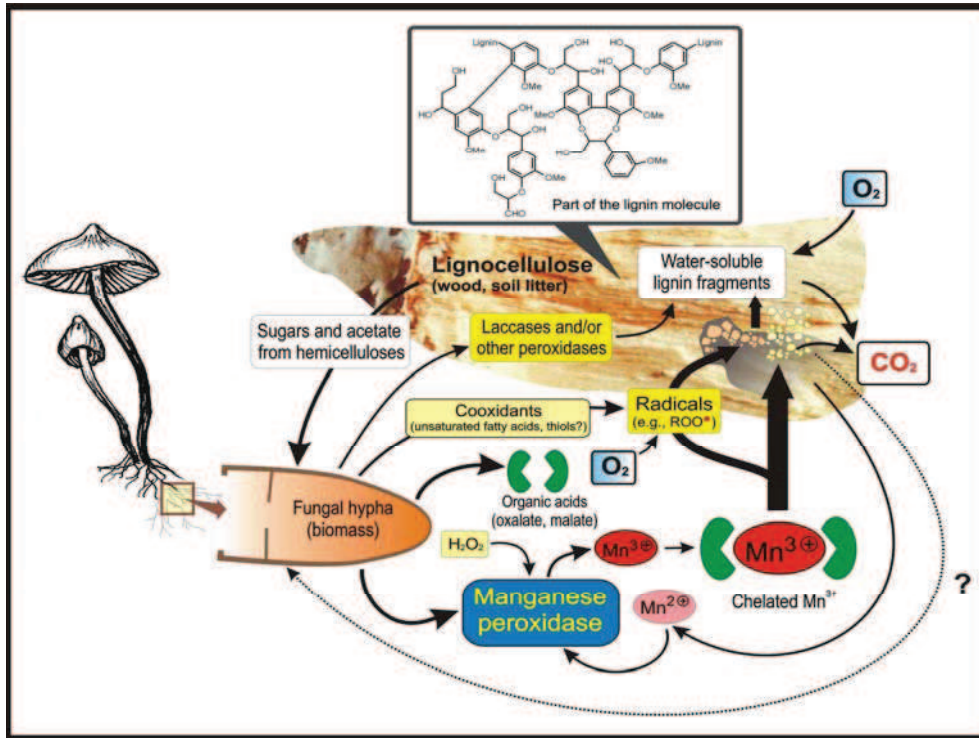
Figure 6 : Système de dégradation du bois par les champignons ligninolytiques (Hofrichter, 2001). Pour dégrader le bois, les champignons excrètent: 1- des oxydants qui vont générer des radicaux très réactifs 2- des manganèse peroxydases qui vont générer du Mn^{3+} qui va se complexer avec des acides organiques excrétés par le champignon. Ce complexe très réactif pourra agir sur la 3- d'autres enzymes telles que des laccases ou des peroxydases (ex: lignine peroxydases).
