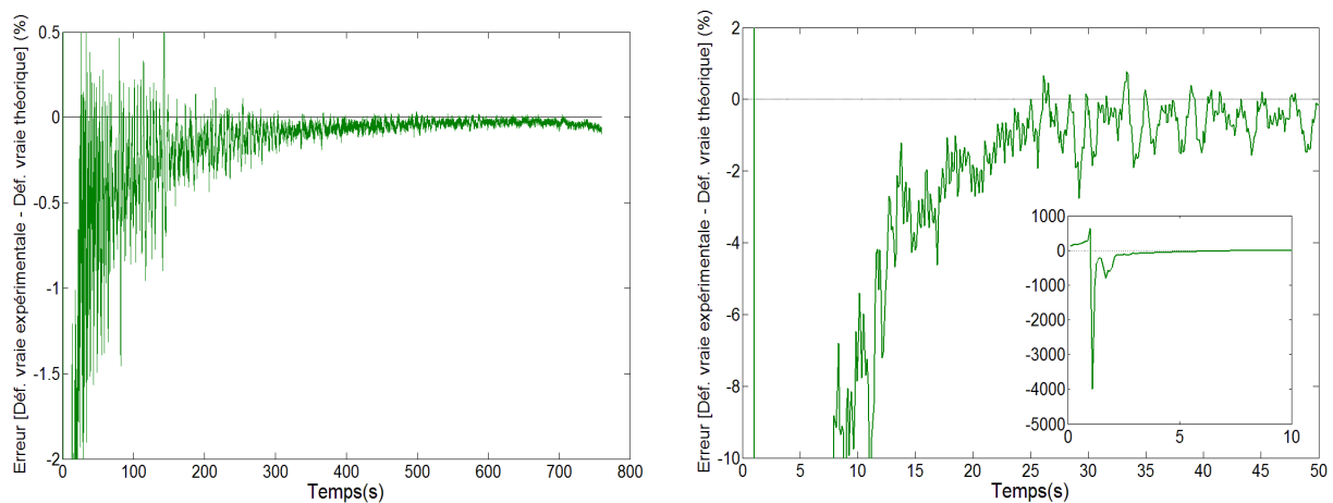
Fig. A1.8 : Ecart entre la déformation vraie longitudinale mesurée et la commande imposée pour le pilotage (essai de traction à vitesse de déformation constante \dot{\varepsilon}_{11} = 2.5 \cdot 10^{-3} \text{ s}^{-1} ).
