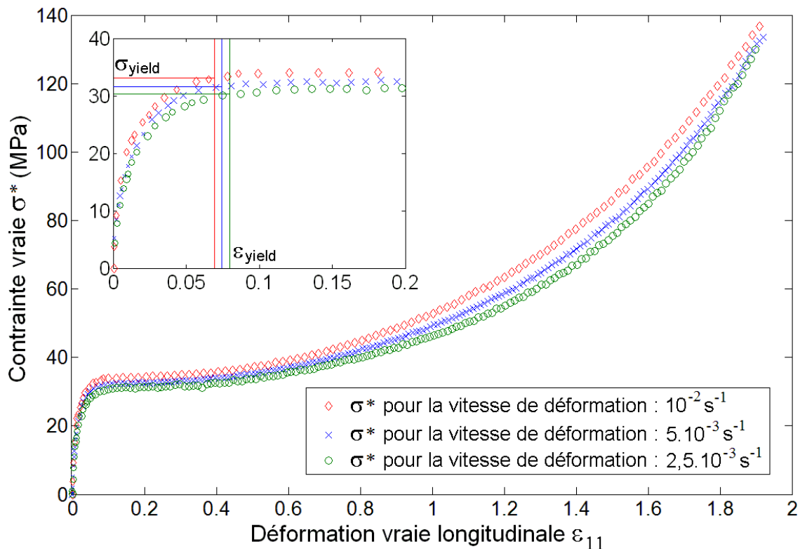
Fig. B.13 : Courbes de traction \sigma^*(\epsilon_{11}) pour l'échantillon A_{//} à différentes vitesses de déformation.
