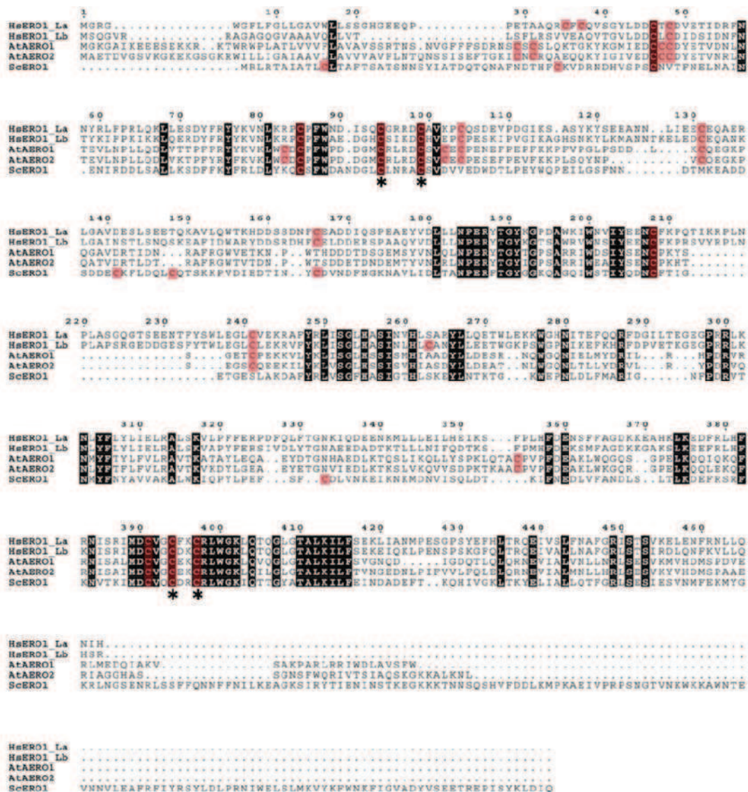
Figure 42. Alignement de séquences primaires des protéines EROs issues de différents organismes. Sont représentées les séquences des deux isoformes des protéines ERO humaine HsERO1-La et HsERO1-Lb (accessions NP_055399.1 et NP_063944.3, respectivement). Les deux isoformes d' Arabidopsis AtAERO1 et AtAERO2 (accessions AT1G72280 et AT2G38690, respectivement), et la protéine ERO1 de Saccharomyces (accession D6W0F5) sont présentées. Les acides aminés strictement conservés sont surlignés en noir et les résidus cystéinyles en rouge. Les astérisques indiquent les résidus cystéinyles essentiels à l'activité de la protéine. La numérotation est différente de celle reportée dans le texte du à l'alignement de séquence.
