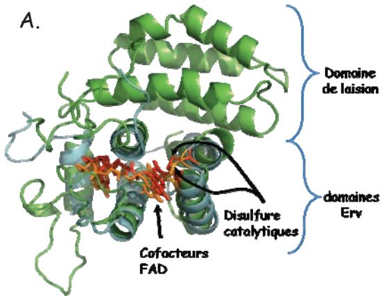
Figure 39. Comparaison du domaine Erv de la protéine humaine Qsox1 et de la protéine AtErv1. A. Superposition des structures tridimensionnelles du fragment HRR/Erv de la protéine HsQsox1 (vert, PDB 3LLk) et de la protéine Erv1 d' Arabidopsis (bleu pâle, PDB 2HJ3). Les cofacteurs FAD ainsi que les ponts disulfure catalytiques CRDC et CREC sont représentés en bâtonnets rouge pour HsQsox1 et orange pour AtErv1. B. Alignement de séquences des protéines AtErv1 et du fragment Erv de la protéine HsQsox1. Les acides aminés surlignés en noir sont conservés. Les structures secondaires des protéines AtErv1 et HsQsox1 sont respectivement représentées en partie haute et basse de l'alignement de séquence.
