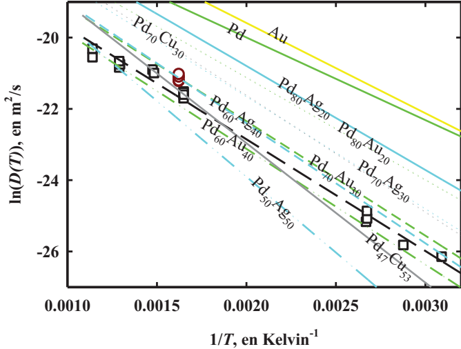
Figure 23 – Diagramme représentant l’évolution du logarithme népérien de D(T) en fonction de l’inverse de la température pour la membrane Au-Pd de la ligne à hydrogène n°1 déterminé dans cette étude (droite en noir, qui est l’interpolation des valeurs expérimentales, représentée par des carrés noirs) comparé à d’autres études (Sonwane et al, 2006 : pour Pd pure, Pd-Au et Pd-Ag, représentée par les droites en vertes et bleues respectivement ; Kamakoti et al., 2005 : pour Pd-Cu, droites en grises ; Zvesdin et Belyakov, 1967 : pour Au, droite en jaune). (Ligne à hydrogène n°2, ronds en rouges).
