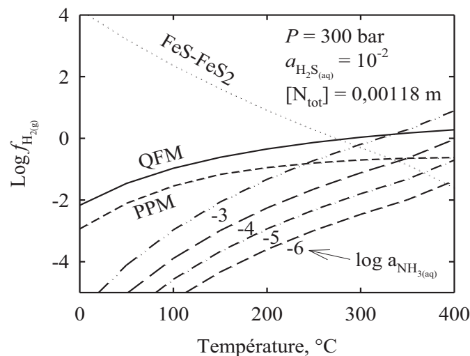
Figure 2 – Diagramme d'équilibre de formation de l'ammoniac (NH 3 ) à partir de N 2 et H 2 (équation 6)
