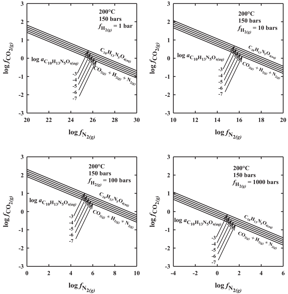
Figure 40 – Représentation des droites d'équilibre \log f_{\text{CO}_2(\text{g})} = f(\log f_{\text{N}_2(\text{g})}) caractéristiques de la réaction de transformation de l'adénosine en \text{CO}_2 , \text{N}_2 et \text{H}_2 selon l'équation (112) :
