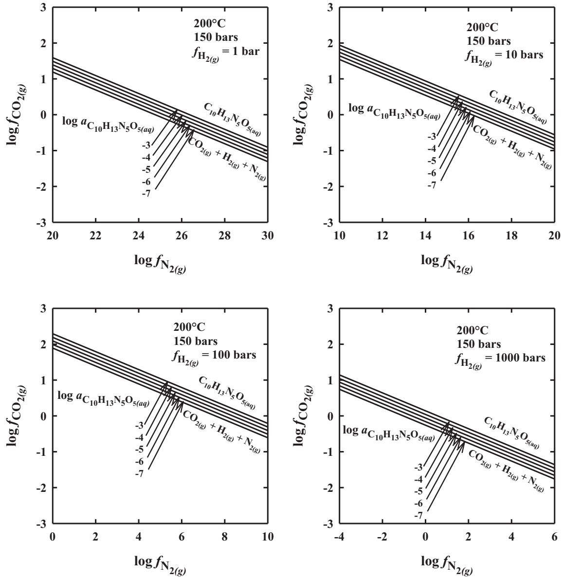
Figure 44 – Représentation des droites d'équilibre \log f_{\text{CO}_2(\text{g})} = f(\log f_{\text{N}_2(\text{g})}) caractéristiques de la réaction de transformation de la guanosine en \text{CO}_2 , \text{N}_2 et \text{H}_2 selon l'équation (124) :
