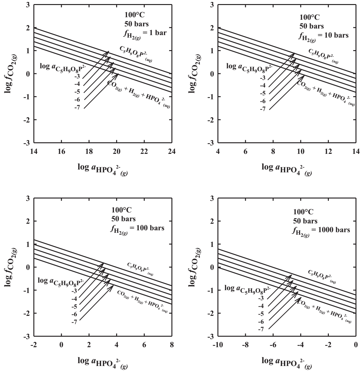
Figure 52 – Représentation des droites d'équilibre \log f_{\text{CO}_2(\text{g})} = f(\log a_{\text{HPO}_4^{2-}(\text{aq})}) caractéristiques de la réaction de transformation du ribose-5-phosphate en \text{CO}_2 , \text{N}_2 et \text{H}_2 selon l'équation (148) :
