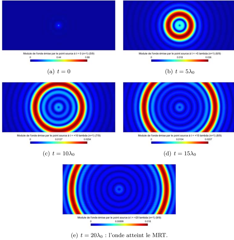
FIGURE 3.23 – Module de l'onde \mathcal{U}_E émise par le point source sur le domaine de calcul \Omega_e à différents instants t et dans un milieu homogène ( n = 1 ). La bande de fréquences utilisée étant [k_0 - k_0/5, k_0 + k_0/5] . Pour une meilleure lisibilité, l'échelle est adaptée à chaque pas de temps.
