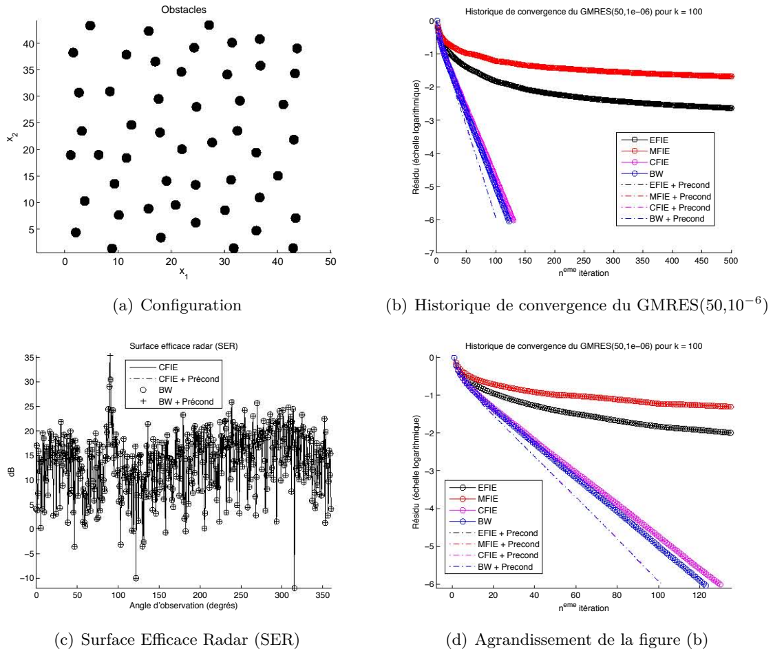
FIGURE 4.5 – La figure (a) présente les M = 50 disques unitaires placés aléatoirement dans la boîte [0, 45]^2 , tels que la plus petite distance b_{pq} entre les centres de deux obstacles \Omega_p^- et \Omega_q^- vérifie b_{pq} \geq 3(= 3a) . Sur la figure (c), nous représentons la section efficace radar obtenue pour k = 100 avec la CFIE (préconditionnée ou non) et l'équation intégrale de Brakhage-Werner preconditionnée par la diffraction simple. Enfin, les figures (b) et (d) présentent l'historique de convergence du GMRES(50, 10^{-6} ) pour les quatre équations intégrales considérées et leurs versions preconditionnées par la diffraction simple (symbolisées par "+ Precond").
