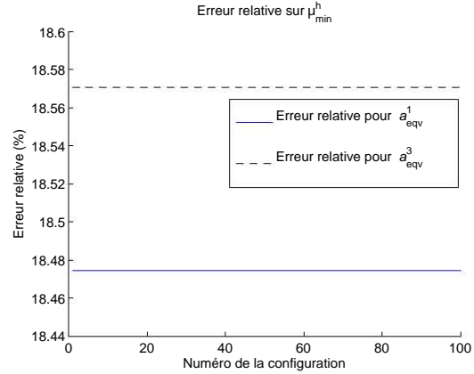
(b) Erreur relative sur \mu_{min}^h
