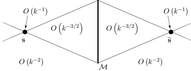
FIGURE 3.6 – Schéma récapitulatif des différentes zones de décroissance du module de u_{RE}
