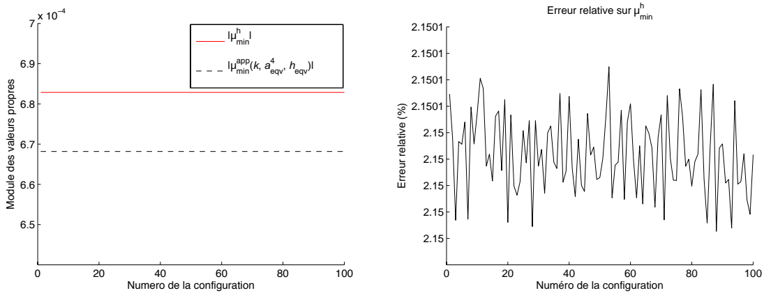
(a) Comparaison entre le module de la plus petite valeur propre (en module) et son estimation (b) Erreur relative sur le module de \mu_{\min}^h
