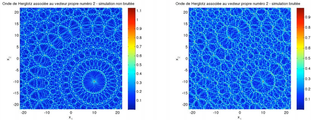
(d) Module de l'onde de Herglotz associée au deuxième vecteur propre de \mathbb{T} (e) Simulation bruitée - Module de l'onde de Herglotz associée au deuxième vecteur propre de \tilde{\mathbb{T}}
