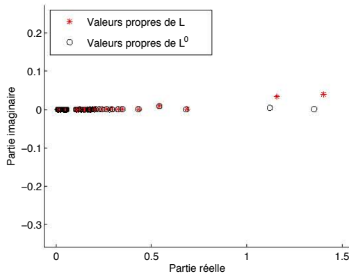
(c) Agrandissement de la figure (b) au niveau de l'origine
