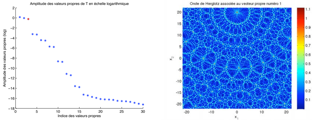
(a) Valeurs propres de \mathbb{T} (échelle logarithmique) (b) Module de l'onde de Herglotz associée au premier vecteur propre de \mathbb{T}
