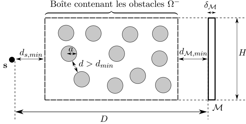
FIGURE 3.15 – Schéma récapitulant les différentes distances intervenant dans la géométrie du domaine. En pratique, les distances d_{s,\min} , d_{M,\min} et d_{\min} sont égales à \lambda/5 , très petites devant D et H . De plus, les obstacles sont petits, de rayon a = \lambda/5 et en grand nombre ( M = 400 ). Un exemple d’une réalisation de milieu est proposée sur la figure 3.10.
