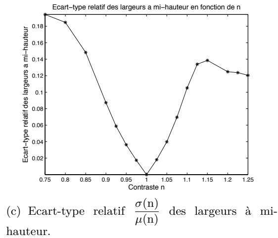
FIGURE 3.18 – Moyenne \mu , écart-type \sigma et écart-type relatif \sigma/\mu des largeurs à mi-hauteur pour 100 configurations d'obstacles en fonction du contraste n .
