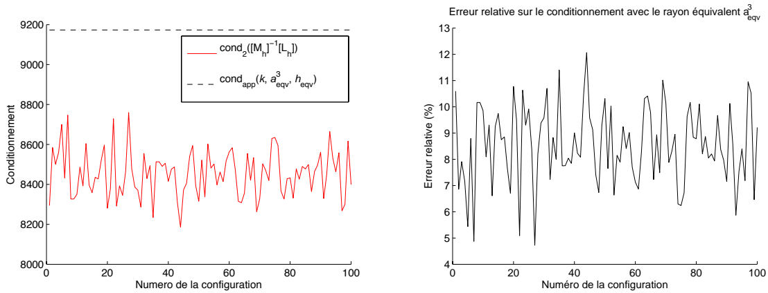
(a) Comparaison entre le conditionnement exact et approché (b) Erreur relative sur le conditionnement
