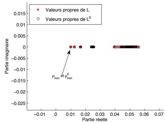
(d) Agrandissement au niveau des valeurs propres de plus petit module \mu_{min} et \mu_{min}^0
