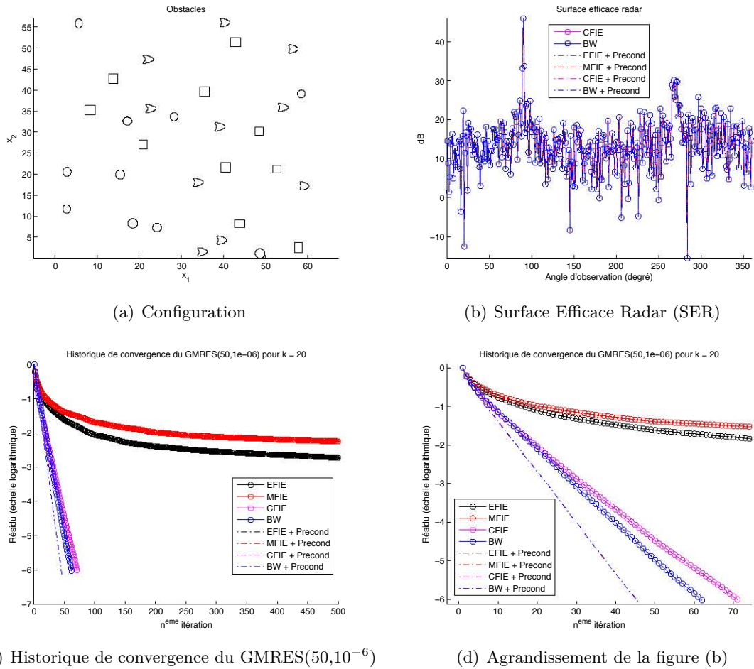
FIGURE 4.7 – La figure (a) présente les M = 30 obstacles des trois formes proposées : ellipses, rectangles et cerfs-volants. Les objets sont disposés aléatoirement dans la boîte [0, 60]^2 , tels que la plus petite distance b_{pq} entre les centres de deux obstacles \Omega_p^- et \Omega_q^- vérifie b_{pq} \geq 3 . Sur la figure (b), nous représentons la section efficace radar obtenue pour k = 20 avec la CFIE et l'équation de Brakhage-Werner (préconditionnées et non preconditionnées). Enfin, les figures (c) et (d) présentent l'historique de convergence du GMRES(50,10 -6 ) pour les quatre équations intégrales considérées et leurs versions preconditionnées par la diffraction simple (symbolisées par “+ Precond”).
