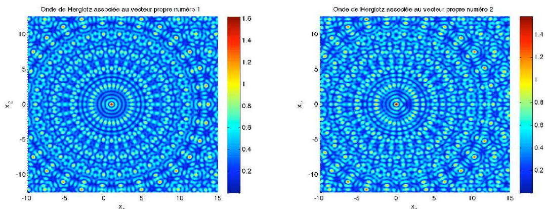
(b) Module de l'onde de Herglotz associée au premier vecteur propre de \mathbb{T}
