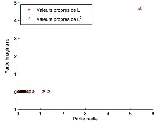
(b) Valeurs propres de \mathbb{L} et de \mathbb{L}^0
