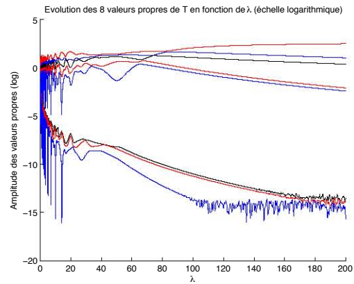
(b) Echelle logarithmique de l'amplitude des 8 valeurs propres de T
