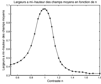
(a) Largeurs à mi-hauteur des champs moyens
