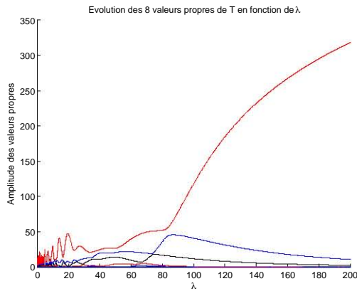
(a) Amplitude des 8 valeurs propres de T
