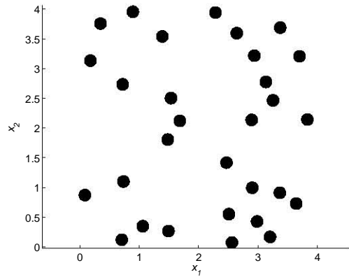
(a) Disposition des obstacles
