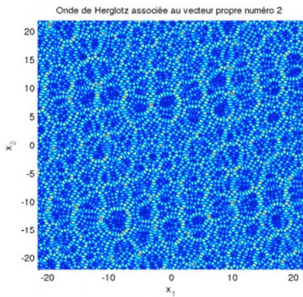
(c) Module de l'onde de Herglotz associée au deuxième vecteur propre de \mathbb{T}
