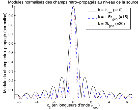
FIGURE 3.13 – Modules normalisés des champs rétro-propagés calculés au niveau de la source pour k = k_{\text{geo}} (= 10) , k = 1.5k_{\text{geo}} (= 15) et k = 2k_{\text{geo}} (= 20) . En abscisse est indiqué la coordonnée x_2 en longueurs d’onde \lambda_{\text{geo}} . Le lobe central se resserre avec l’augmentation de la longueur d’onde k .
