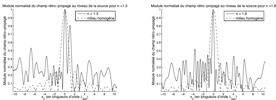
(a) n = 1.3 : présence de pics secondaires.
