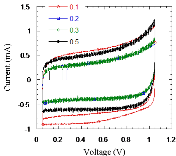
Fig. 9 : Courbes de voltammétrie cyclique à 2mV/s, pour différents rapports molaire P/F.
