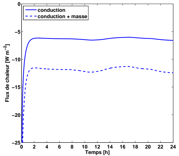
(b) Flux de chaleur en hiver
