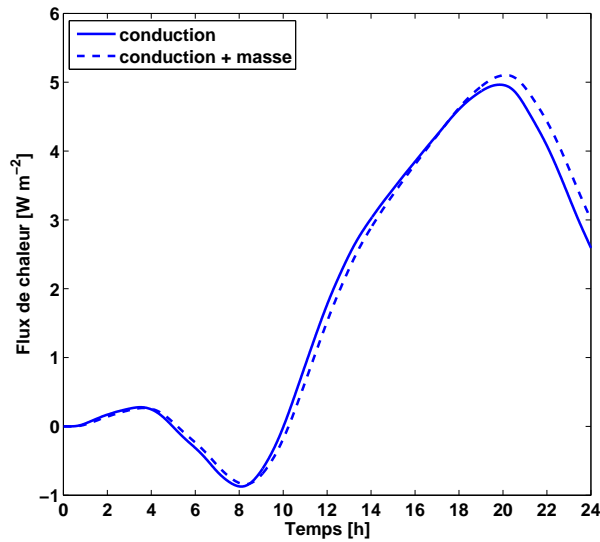
(a) Flux de chaleur en été
