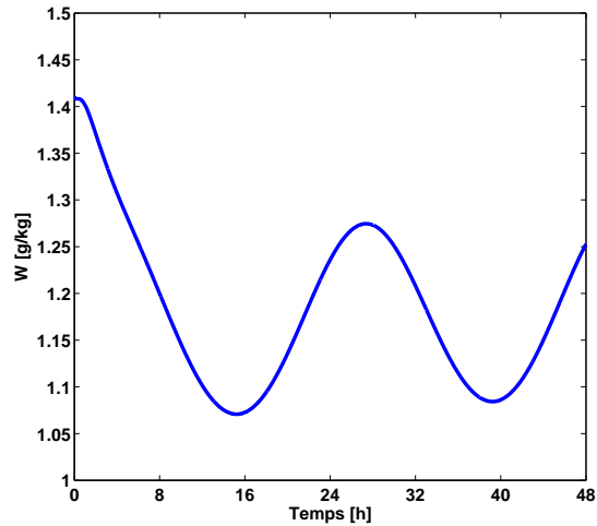
FIG. 5.10 – Fraction massique de vapeur d’eau au centre de la lame d’air
