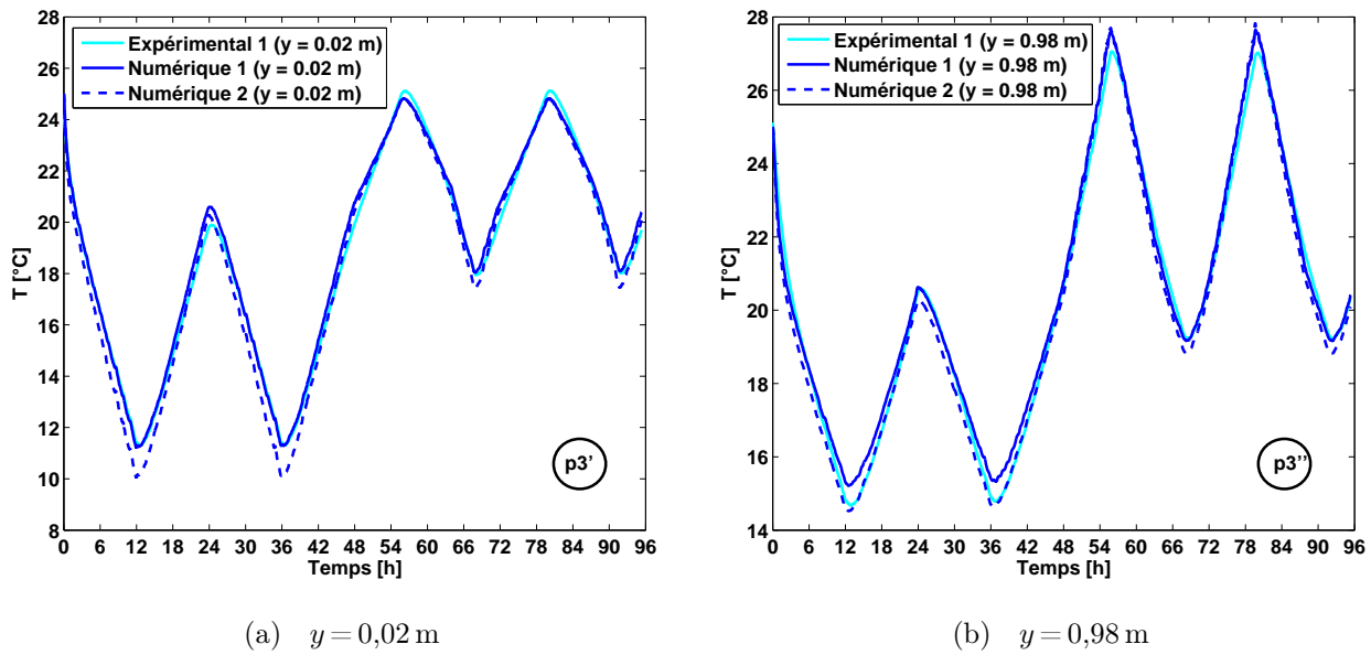
FIG. 7.16 – Évolutions de températures à y = 0,02 \text{ m} et y = 0,98 \text{ m} dans la lame d'air
