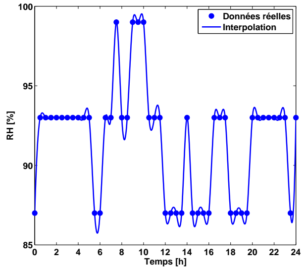
(b) Humidité relative extérieure
