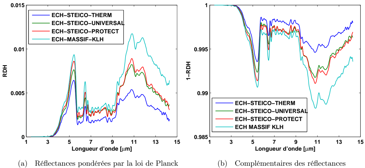
FIG. 6.43 – Mesures de réflectances pondérées par la loi de Planck
