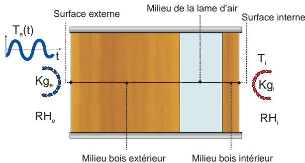
FIG. 5.7 – Deuxième cas test : couplage entre codes avec une paroi soumise à une évolution sinusoïdale de température extérieure
