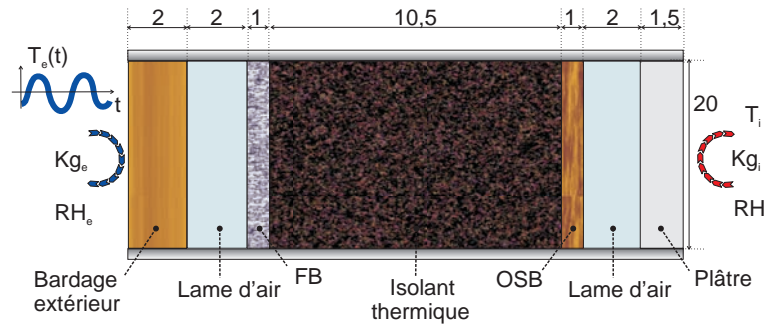
FIG. 4.14 – Modèle réel de paroi
