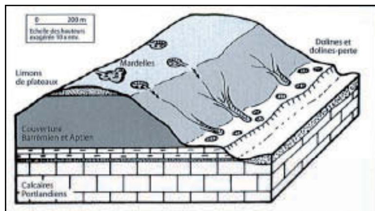
Figure 4.17 - Bloc diagramme schématique montrant l'association des mardelles en position sommitale et des dolines en pied de versant en Woëvre (Meuse, Lorraine). Figure extraite de S. Jaillet (2005).
