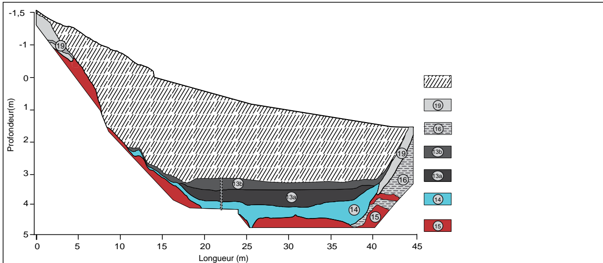
Figure 3.5 - Photographie et schéma de la coupe de la mardelle de Bisping (BIS) réalisée lors des fouilles archéologiques de l'INRAP en 2009 et des Unités Stratigraphiques (US) identifiées sur le terrain avec Stéphanie Goepf et Etienne Dambrine.
