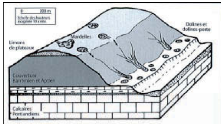
Figure 4.17 - Bloc diagramme schématisant l'association des mardelles en position sommitale et des dolines en pied de versant en Woëvre (Meuse, Lorraine). Figure extraite de S. Jaillet (2005).
