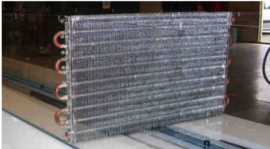
figure 4.2 - Photographie de l'échangeur de chaleur
