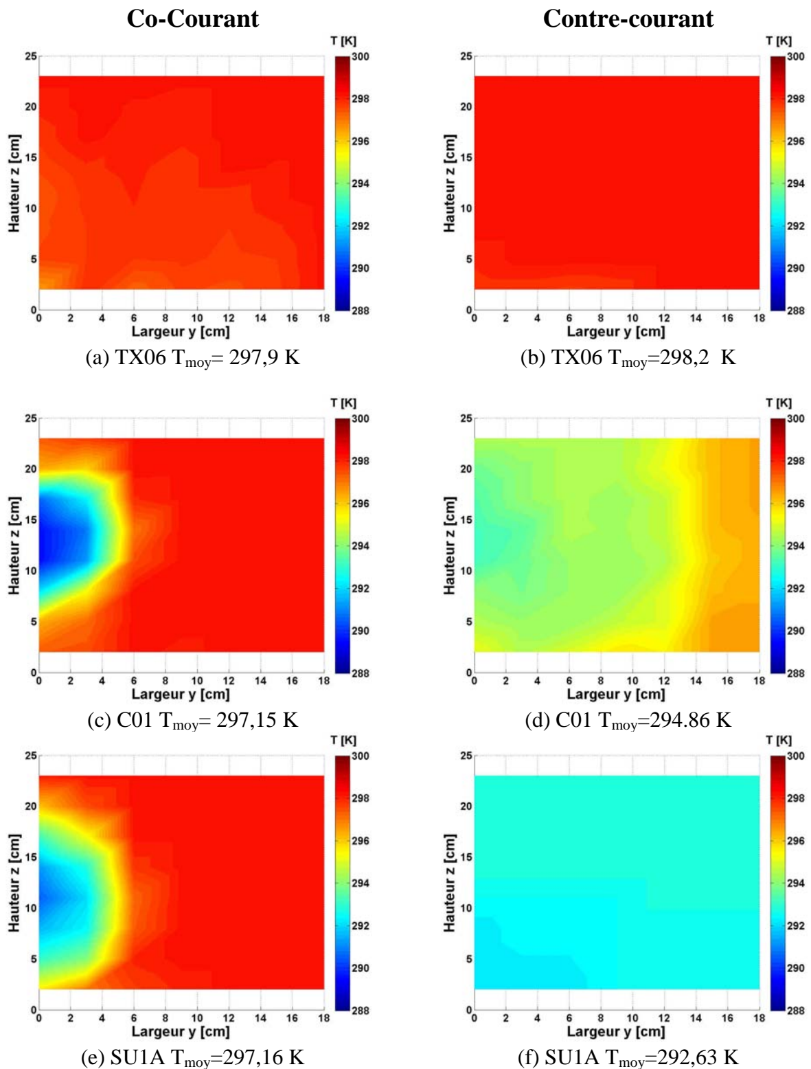
figure 4.31 - Température de l'écoulement d'air en fonction de la buse et du sens d'injection du spray
