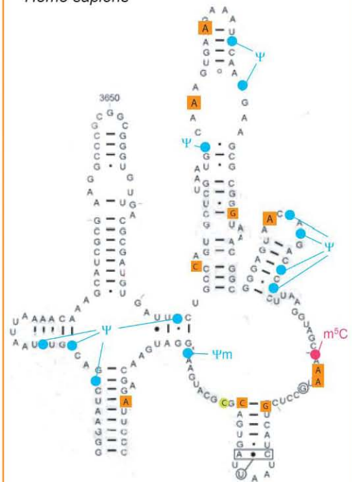
Homo sapiens
