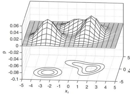
Fig. 9.13 – Surface d'une densité de probabilité en 2D d'un modèle de mélange de gaussiennes à trois composantes et les surfaces d'équiprobabilités correspondantes.
