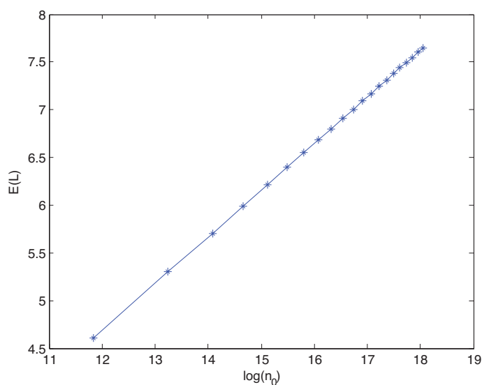
FIGURE 4.7 – Variation de E(L) en fonction de \log(n_0) , avec m = 3 , q = 0.6 , \mu = 1 et r = 0.4 .
