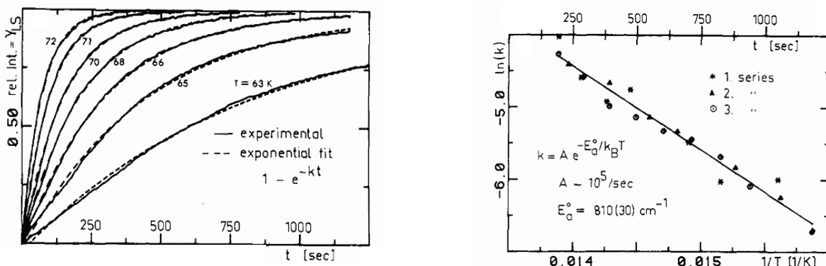
Figure II.10 À gauche : Courbes de relaxation mono-exponentielles du composé [\text{Fe}_{0.1}\text{Zn}_{0.9}(\text{ptz})_6](\text{BF}_4)_2 en fonction de la température. À droite : Tracé d'Arrhenius \ln k_{\text{HB}} vs. 1/T . [II.30]
