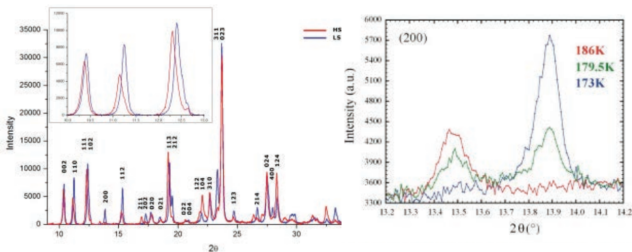
Figure II.15 Spectres de diffraction sur poudre du composé [\text{Fe}(\text{phen})_2(\text{NCS})_2] [II.51]. À gauche : Superposition de deux spectres de diffraction pour l'état BS (bleu) et HS (rouge). Encart : déplacement en 2\theta pour les trois premiers pics. À droite : Évolution du profil de diffraction dans la région de la réflexion (200) en fonction de la température dans le domaine de la transition thermique
