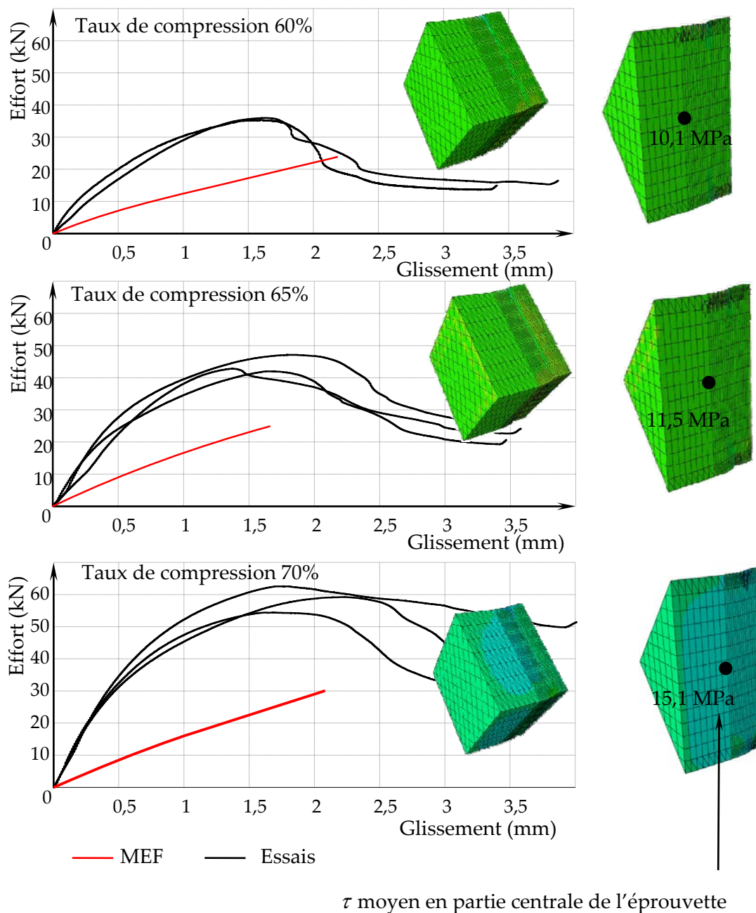
Figure 96 : Comportement expérimental du bois d'épicéa dans le montage de compression cisaillement et réponse du modèle.
