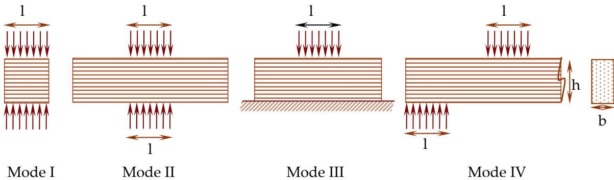
Figure 110 : Différents modes de sollicitation d'éléments bois en compression transversale Blass [56] .
