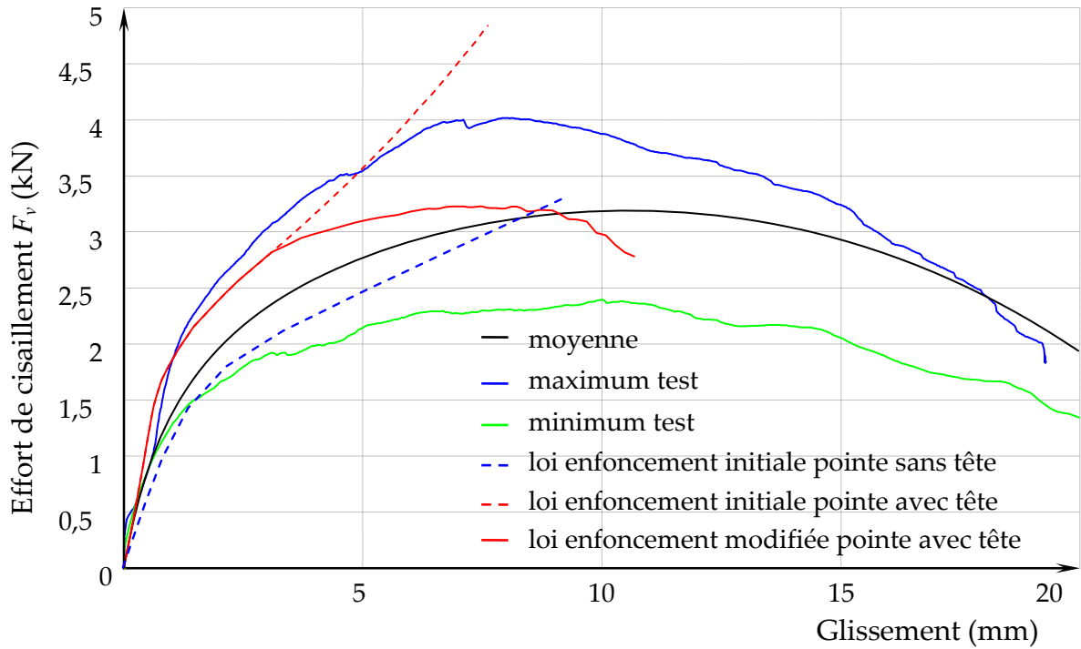
Figure 74 : Comparaison des évolutions effort glissement obtenues en essais et suivant différentes conditions de modélisation (effort pour deux points).
