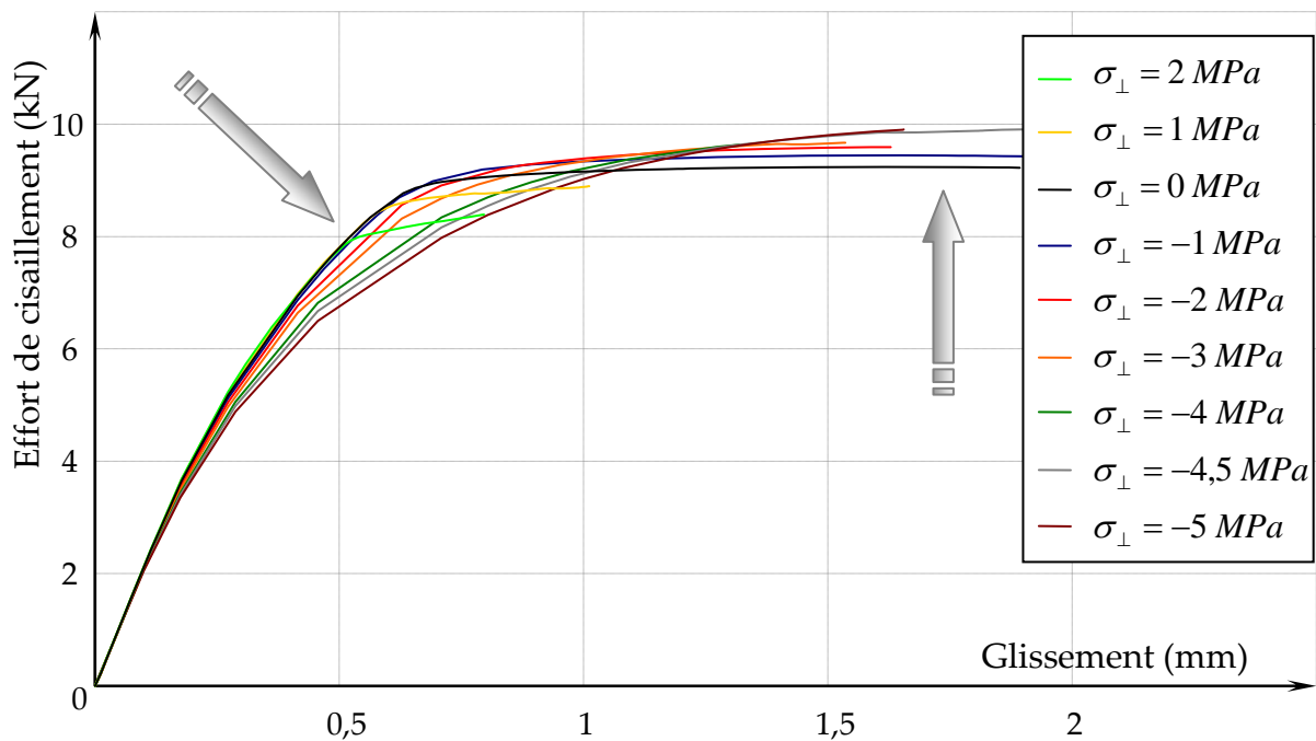
Figure 95 : Évolutions de l'effort de cisaillement en fonction du glissement obtenues par modélisation pour différents états de contraintes transversales.
