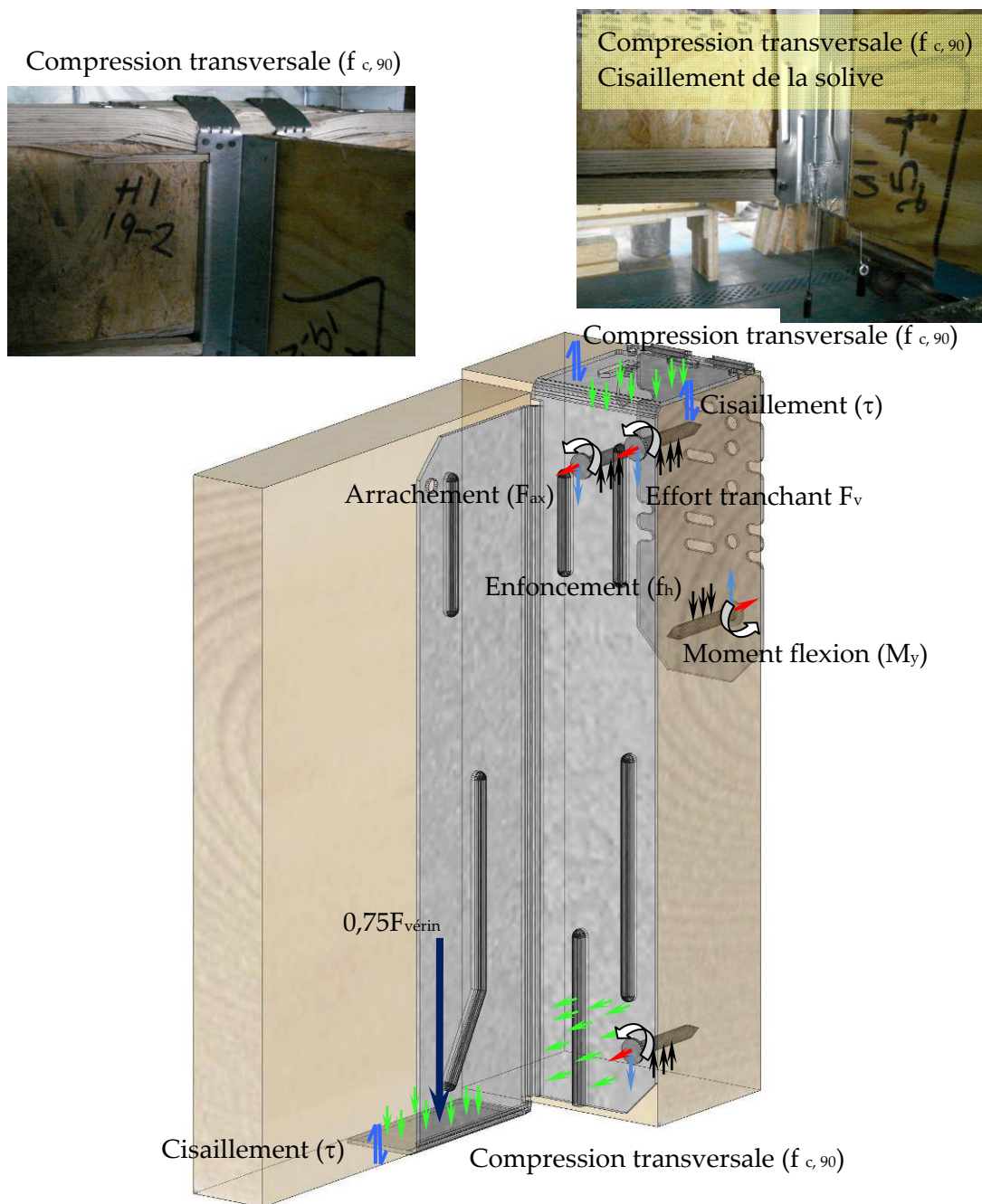
Figure 14 : Efforts intérieurs et modes de rupture les plus observés pour des assemblages du groupe 3 (HII).
