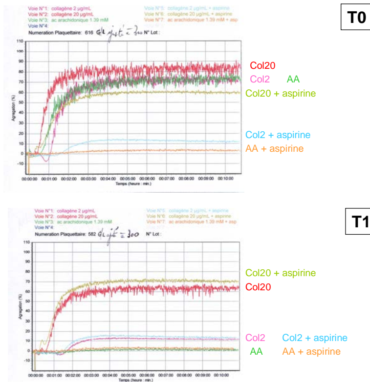
Figure 8 : Exemple de résultat d'agrégométrie photométrique. Patiente traitée, en principe, quotidiennement par 75 mg d'aspirine. T0 : Aucun effet visible de l'aspirine ex vivo. L'agrégation induite par l'AA et Col2 n'est pas inhibée. Inhibition de l'agrégation induite par AA et Col2 après ajout d'aspirine in vitro. T1 : La prise de 300 mg d'aspirine per os permet de voir que l'agrégation induite par AA et Col2 est autant inhibée sans et avec ajout d'aspirine in vitro. Conclusion : réponse plaquettaire à l'aspirine per os visible à T1 sur l'agrégation induite par AA et Col2.
