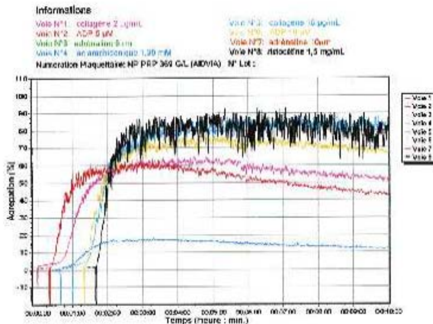
Figure 1 Profil typique d'agrégation plaquettaire photométrique lors d'un traitement par aspirine. Agrégomètre Soderel Medical®. Typical photometric pattern of platelet aggregation in a patient taking aspirin. Agregometer Soderel Medical®.
