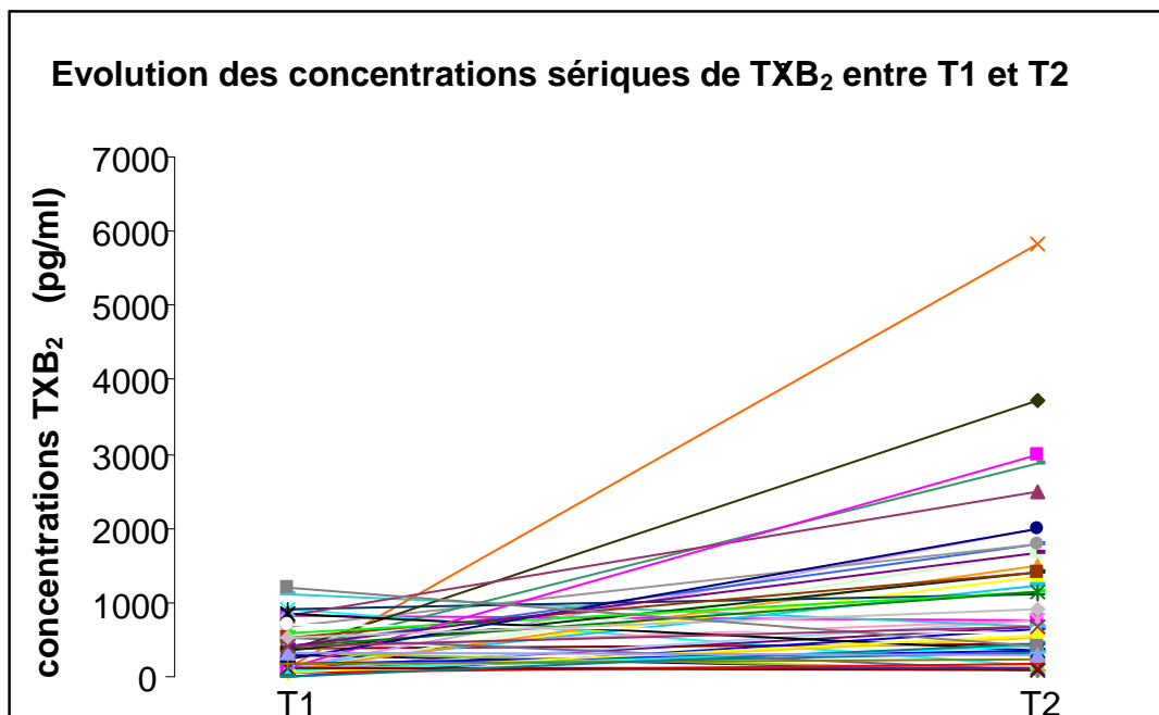
Figure 12 : Evolution des concentrations sériques de TXB 2 entre T1 et T2.
