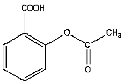
Figure 1 : Formule de l'acide acétylsalicylique
