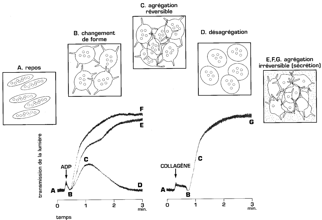
Figure 10 : Exemples de courbes d'agrégation plaquettaire mesurées par agrégométrie photométrique avec pour stimulus l'ADP (à 1,5 \mu M, 2,5 \mu M et 5 \mu M) et le collagène. Extraite de B Boneu, JP Cazenave « Introduction à l'étude de l'hémostase et de la thrombose » 2 e édition (Boehringer Ingelheim France 1997).
