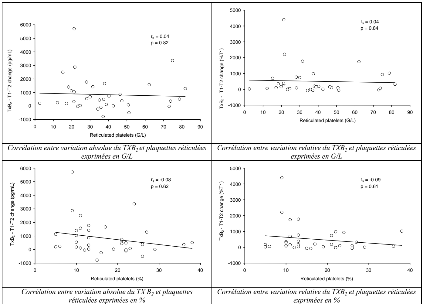
Figure 15 : Recherche d'une corrélation entre les variations de concentrations sériques de TXB_2 et le pourcentage, et la numération de plaquettes réticulées.
