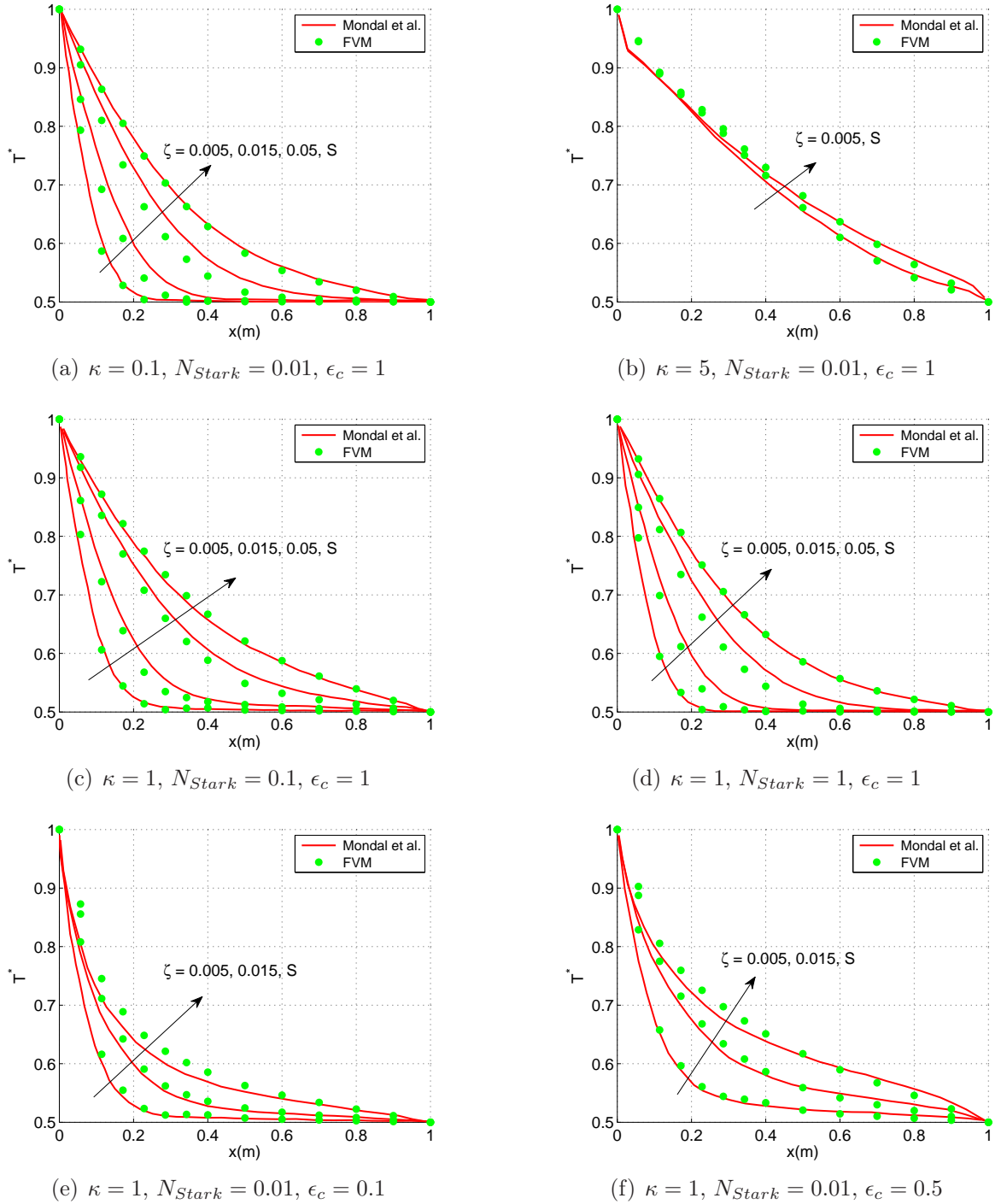
FIGURE 4.15 – Température sur l'axe central du plan médian en z = 0.5 m
