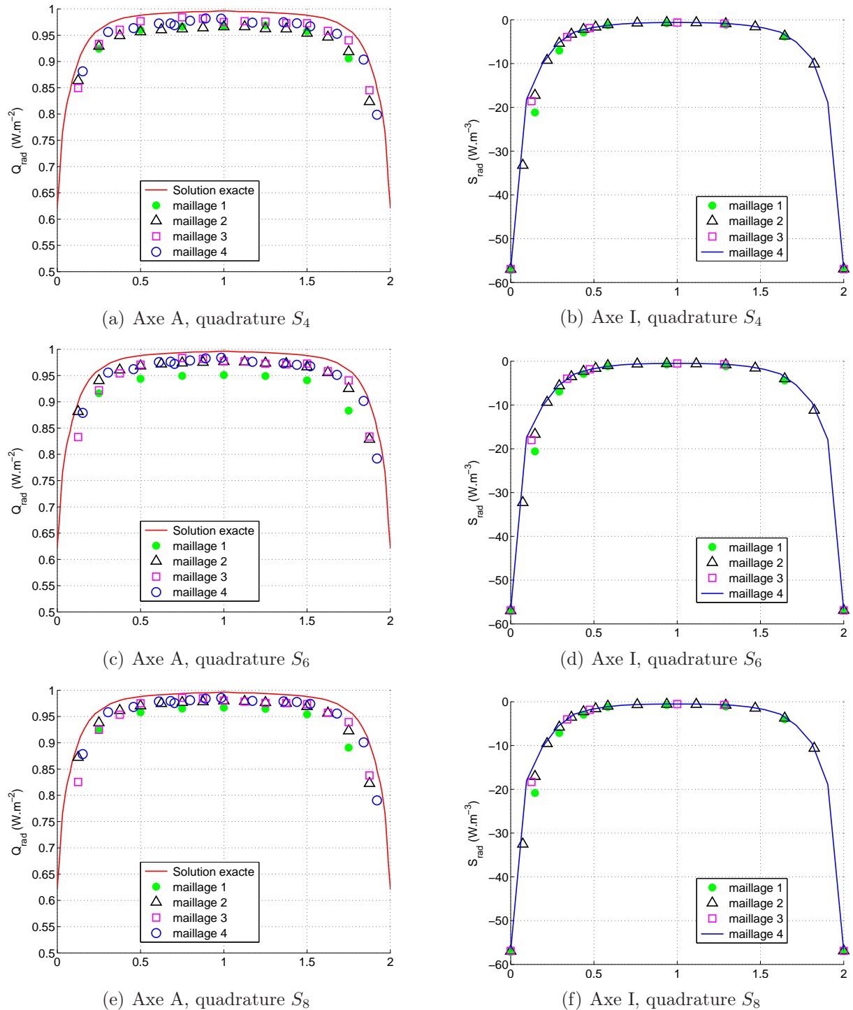
FIGURE 3.27 – Flux radiatif adimensionné (axe A) et terme source radiatif (axe I) pour \kappa = 5 \text{ m}^{-1}
