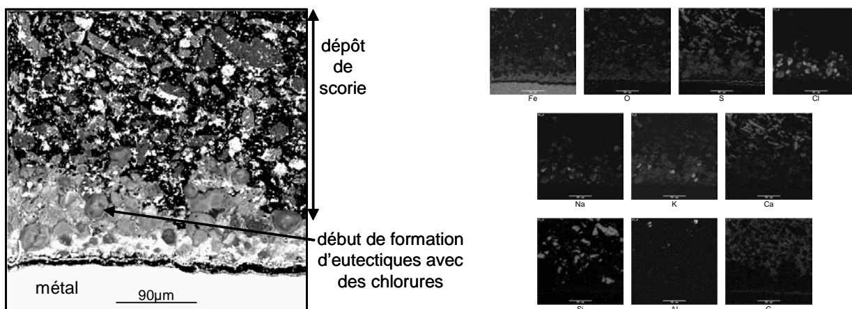
Figure 24 : Photographie MEB et cartographie élémentaire de l'essai réalisé à T_{\text{fumées}} = 450^{\circ}\text{C} , HCl = 200 ppm et \text{SO}_2 = 20 ppm (essai 23-face 90°).
