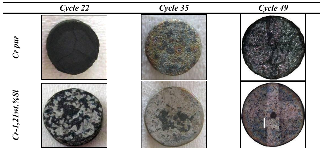
Figure 72 : Aspects extérieurs des échantillons Cr et Cr-1,21wt.%Si au cours d'essais d'oxydation cyclique à 1300°C
