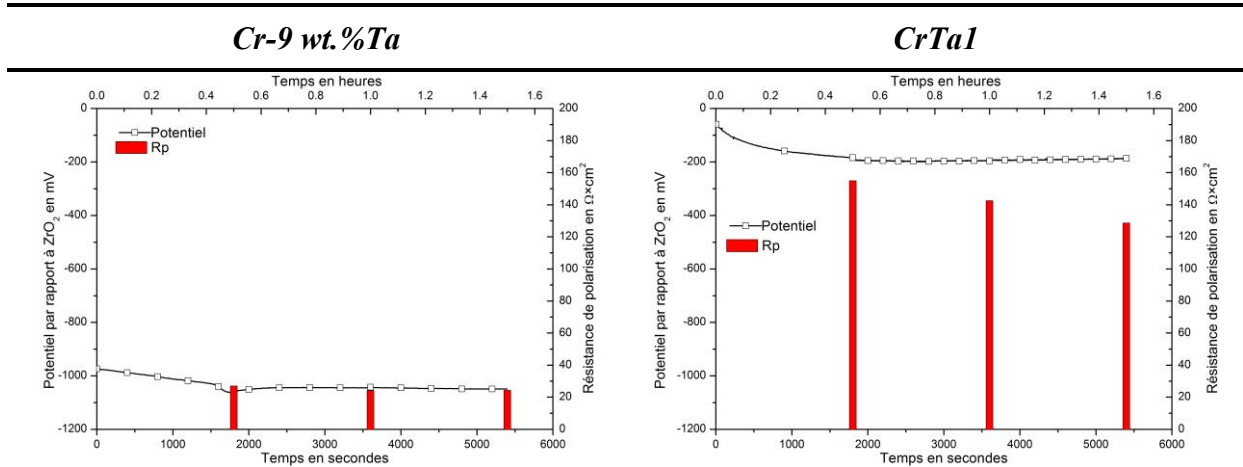
Figure 175 : Suivis de potentiels et des résistances de polarisation des alliages Cr-9 wt.%Ta et CrTa1 préoxydés immergés dans le verre THA à 1200°C
