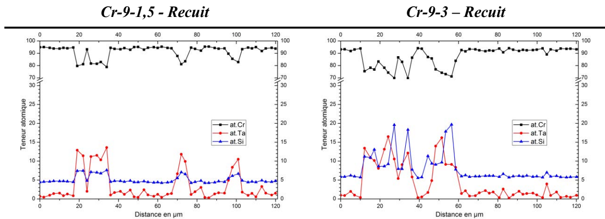
Figure 118 : Profils de concentrations des ternaires Cr-Ta-Si après recuit
