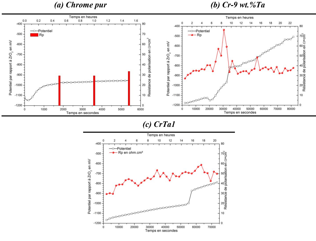
Figure 173 : Suivis de potentiel et de la résistance de polarisation dans le verre THA à 1200°C
