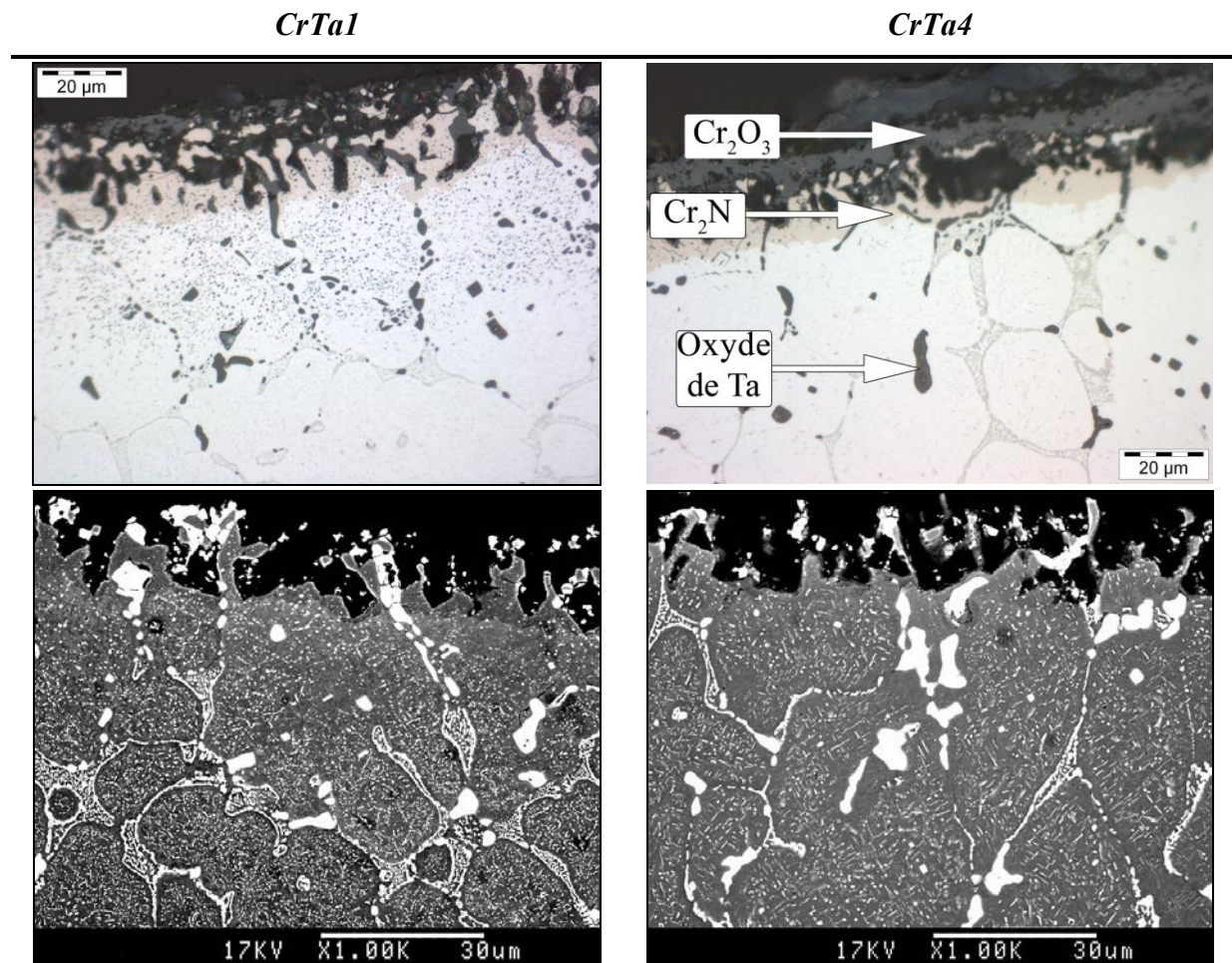
Figure 151 : Observations métallographiques des échantillons CrTa1 et CrTa4 après thermogravimétrie de 20 heures à 1300°C
