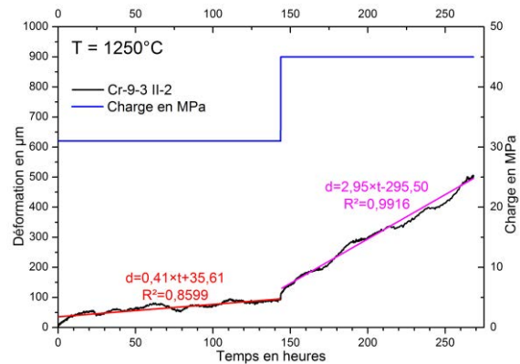
Figure 137 : Courbes de fluage 3 points de l'alliage Cr-9-3 II-2 à 1250°C et sous 31 puis 45 MPa
