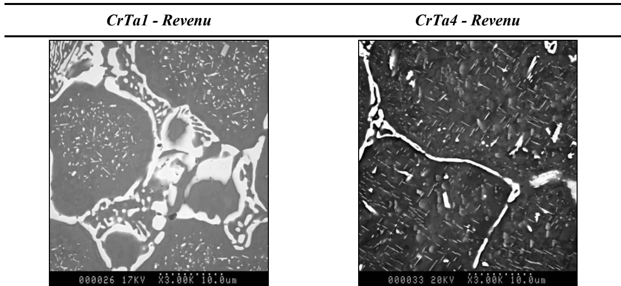
Figure 127 : Observation électronique après revenu des échantillons Cr-Ta-Si substitués au molybdène ou au tungstène
