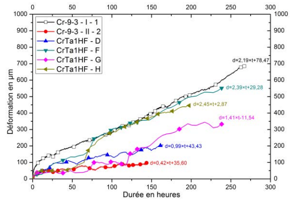
Figure 139 : Comparaison des fluages à 1250°C sous 31MPa des alliages Cr-Cr 2 Ta
