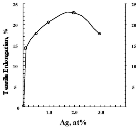
Figure 4 : Evolution de l'allongement maximal en fonction de la teneur en Ag, d'après Gu [30]
