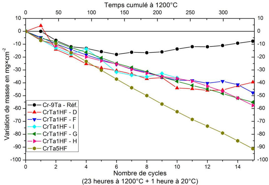
Figure 163 : Variation de masse des échantillons CrTa1 et CrTa5 au cours des essais d'oxydation cyclique à 1200°C
