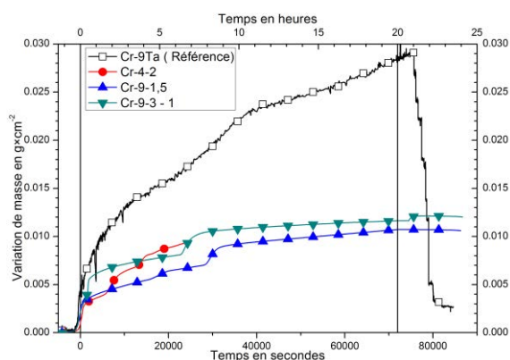
Figure 143 : Thermogrammes d'alliages Cr-Ta-Si oxydés 20 heures à 1300°C
