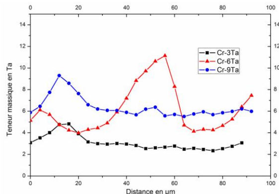
Figure 90 : Profils de concentration des alliages Cr-Ta
