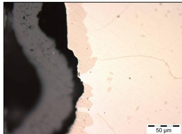
Figure 61 : Influence de l'adhérence de la chromine sur la nitruration du chrome
