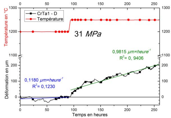
Figure 138 : Courbe de fluage 3 points d'un alliage CrTa1 à 1200°C (en bleu) puis 1250°C (en vert) sous 31 MPa de contrainte
