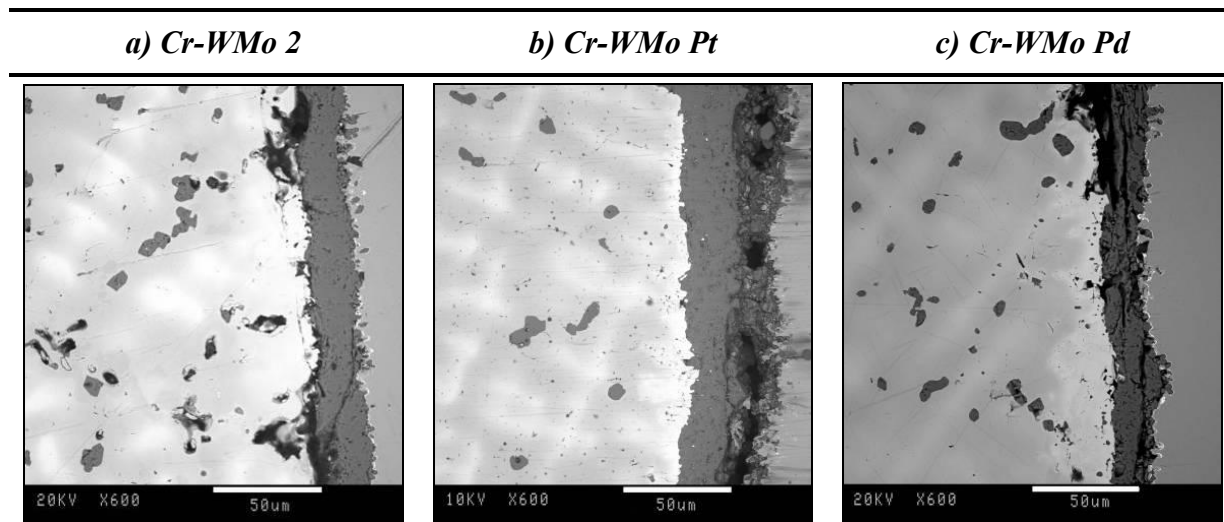
Figure 97 : Image en électrons rétrodiffusés des échantillons oxydés à 1300°C
