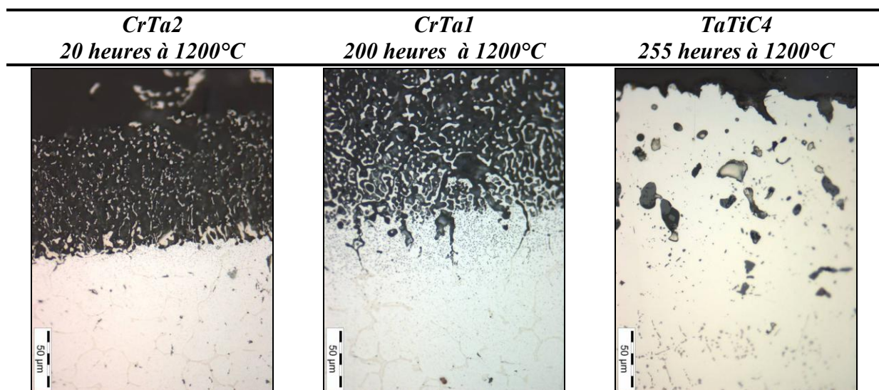
Figure 167 : Faciès de corrosion des alliages Cr-Cr 2 Ta et TaTiC 4 à 1200°C dans du verre industriel C3 à 1200°C
