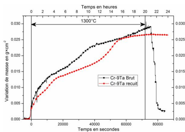
Figure 113 : Courbes thermogravimétriques d'échantillon Cr-9%Ta brut et recuit 24 heures à 1300^\circ\text{C}
