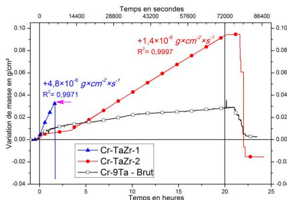
Figure 147 : Thermogrammes des alliages Cr-TaZr-1, Cr-TaZr-2 et Cr-9Ta à 1300°C
