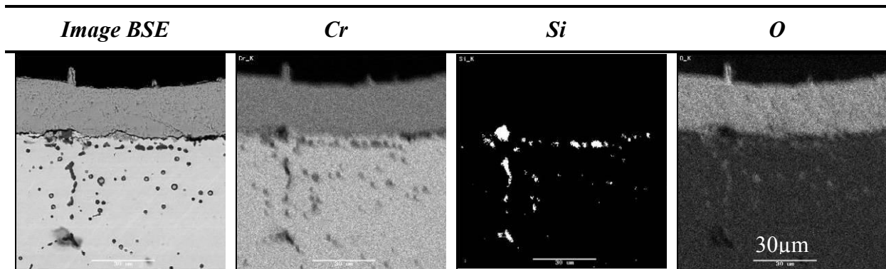
Figure 68 : Image en mode BSE et cartographies EDX de Cr, Si et O de l'échantillon Cr-1,21wt.%Si exposé 20 heures à 1300°C sous air
