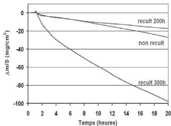
Figure 94 : Oxydation à l'air et à 1300°C de l'alliage brut et recuit à 1300°C
