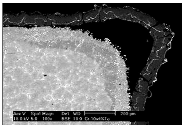
Figure 112 : Cr-10%Ta après 70 heures d'oxydation à 1300^\circ\text{C}
