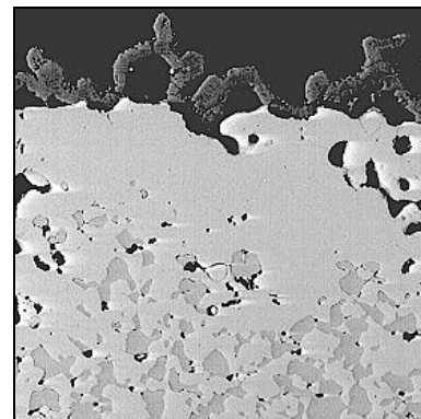
Figure 31 : Faciès d'oxydation d'un alliage Cr-15%Al-Ni après 100 heures à 1300°C, d'après Kessler [4]
