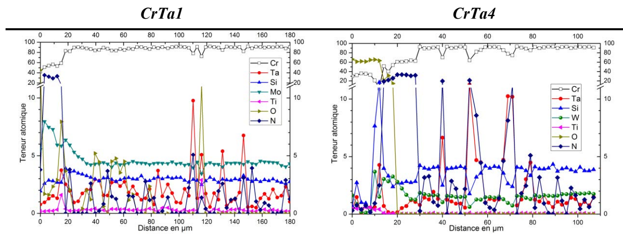
Figure 152 : Profils de concentration obtenus à la microsonde électronique de Castaing des échantillons CrTa1 et CrTa4 après oxydation isotherme de 20 heures à 1300°C
