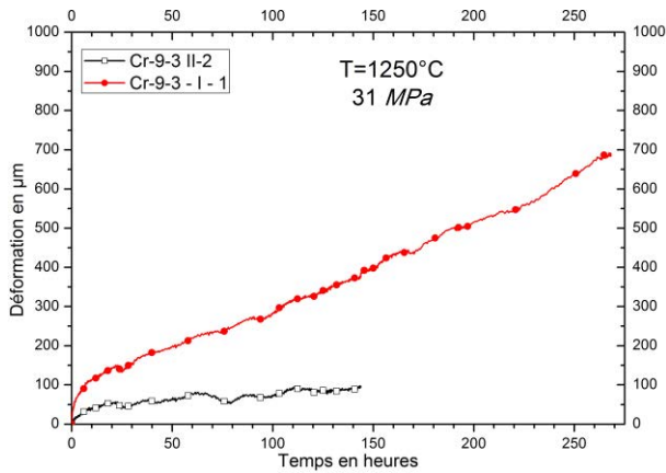
Figure 135 : Influence de l'état métallurgique sur la vitesse de déformation d'alliages Cr-9-3
