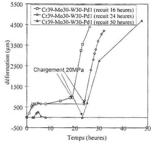
Figure 11 : Courbes de fluage trois points d'alliages Cr-W-Mo-Pd d'après [3]
