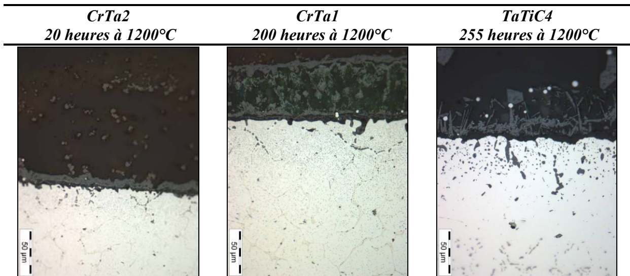
Figure 170 : Faciès de corrosion des alliages Cr-Cr 2 Ta et TaTiC4 à 1200°C immergés dans du verre industriel THA
