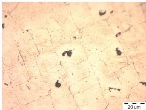
Figure 103 : Mise en évidence des grains de l'alliage Cr-W-Mo Pd-O par une attaque chimique au réactif de Murakami
