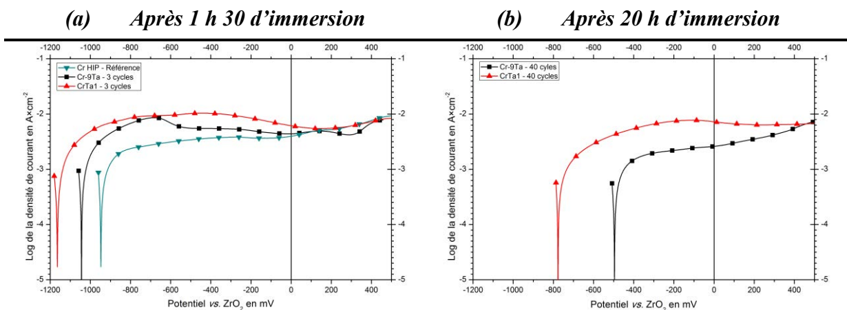
Figure 174 : Courbes Intensité-Potentiel du chrome, de Cr-9 wt.%Ta et de CrTa1 après 1h30 d'immersion (a) et après 20h d'immersion (b) dans le verre THA à 1200°C
