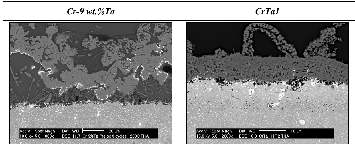
Figure 177 : Micrographies d'alliages Cr-9 wt.%Ta et CrTa1 préoxydés après 2h d'immersion dans du verre THA à 1200°C
