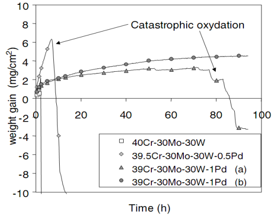
Figure 29 : Influence de la teneur en Pd sur la tenue en oxydation d'alliages Cr-W 30 -Mo 30 -xPd, d'après Diliberto [45]
