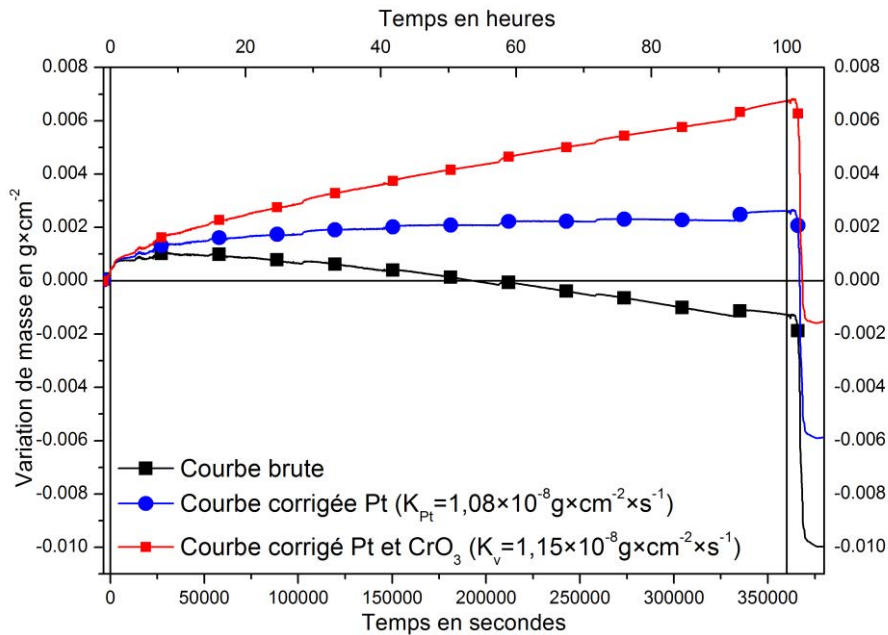
Figure 79 : Thermogramme de la phase \text{Cr}_3\text{Si} brut (en noir), corrigé de la volatilisation de l'appareillage (en bleu) et de la volatilisation \text{Pt}+\text{CrO}_3 (en rouge)
