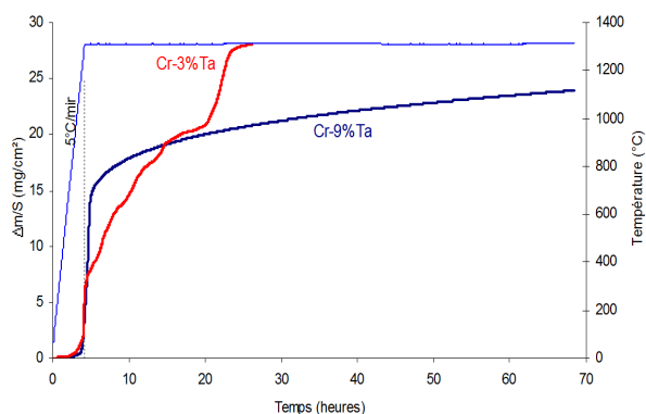
Figure 111 : Essais thermogravimétriques des alliages Cr-3 wt%Ta et Cr-10 wt%Ta à 1300^\circ\text{C} sous air
