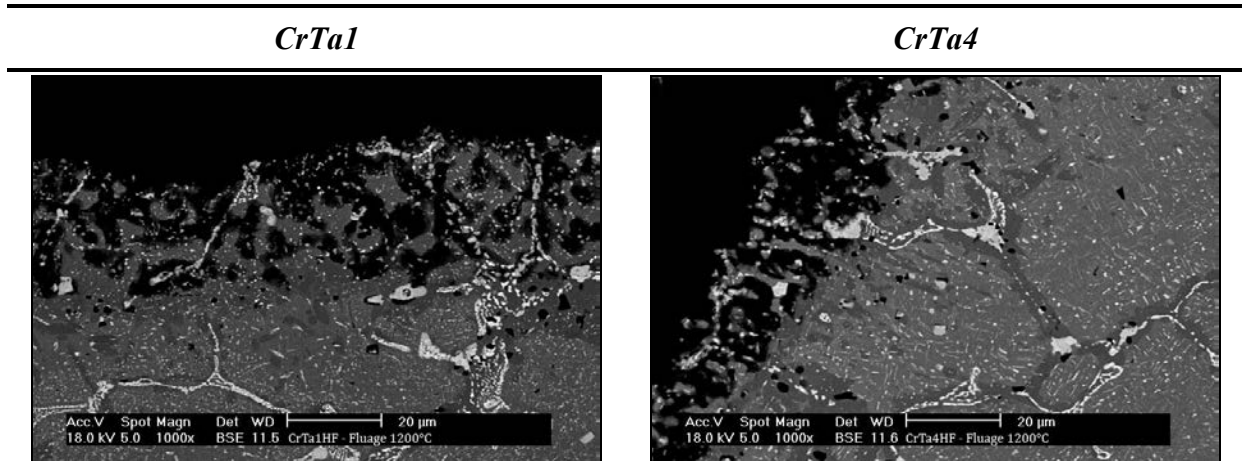
Figure 157 : Images électroniques des coupes transverses des alliages CrTa1 et CrTa4 après essai mécanique de 250h à 1200°C sous 31MPa
