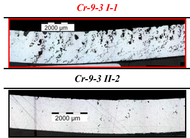
Figure 136 : Mise en évidence de la moins bonne qualité métallurgique de l'échantillon I-1 après essai
