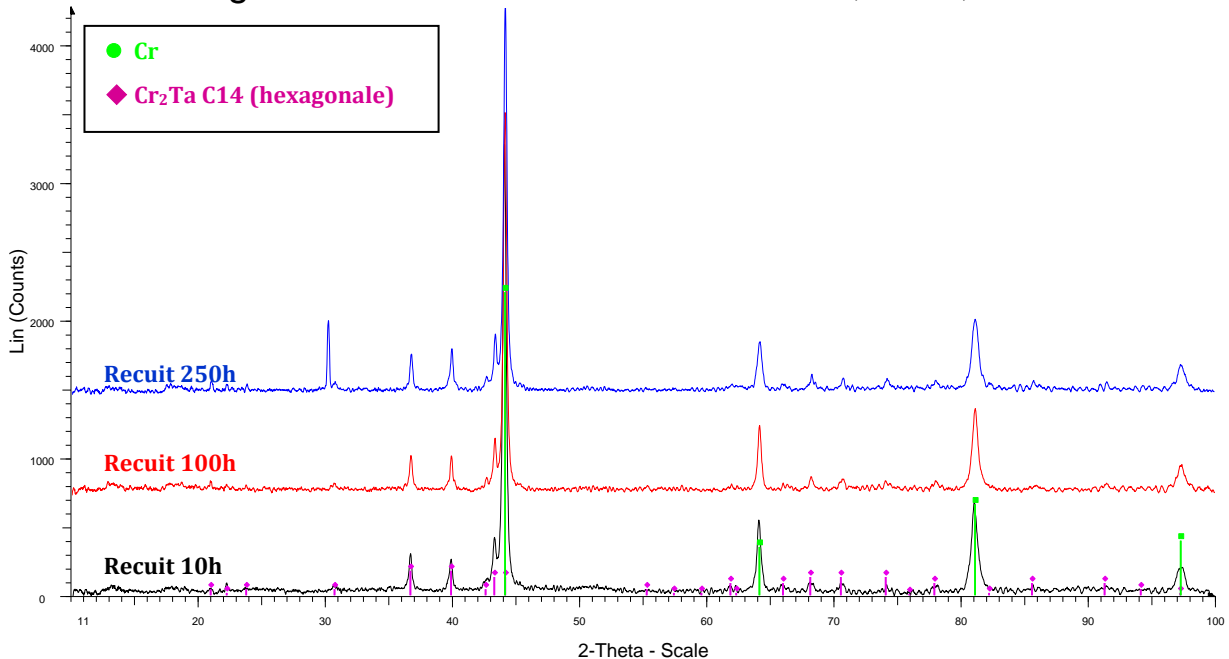
Figure 132 : Différents programmes de l'alliage CrTa1 montrant l'évolution des rates de diffraction de la solution solide de chrome et de la phase Cr 2 Ta.
