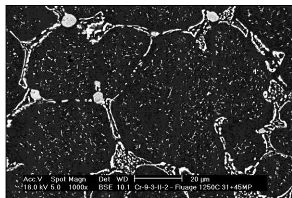
Figure 156 : Exemple de précipitation secondaire, cas de Cr-9-3 II-2
