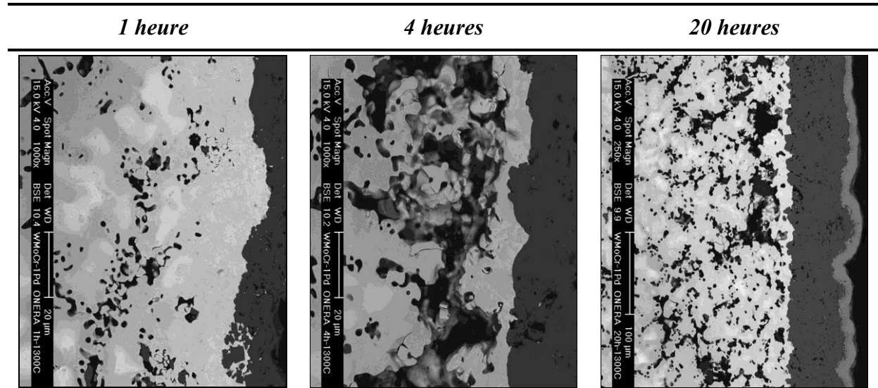
Figure 102 : Alliage Cr-WMo Pd-O à divers temps d'oxydation à 1300°C
