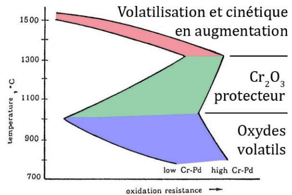
Figure 27 : Résistance à l'oxydation d'alliages W-Cr-Pd en fonction de la température, d'après [86]
