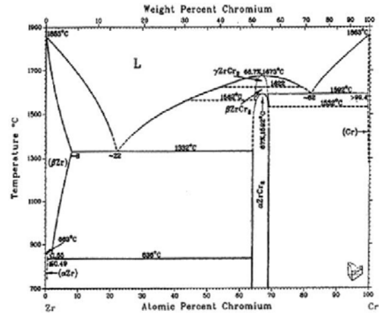
Figure 119 : Diagramme de phases Cr-Zr selon Arias [129]
