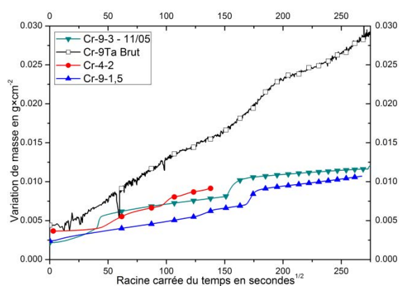
Figure 144 : Mise en évidence des cinétiques paraboliques obtenues
