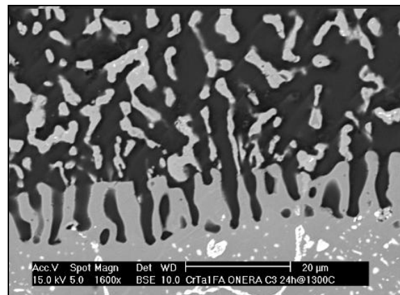
Figure 172 : Echantillon CrTa1 après 24 heures à 1300°C dans du verre C3 – Disparition des phases de Laves.
