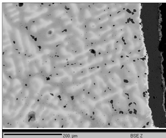
Figure 95 : WMoCr-1 : Image en électrons rétrodiffusés de la plaquette d'oxydation
