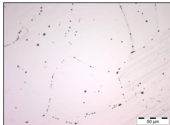
Figure 65 : Micrographie de l'alliage Cr-0,55 wt.% Si à l'issue de l'élaboration
