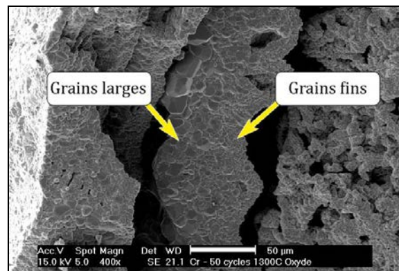
Figure 74 : Vue en coupe d'une couche de chromine développée sur du chrome pur
