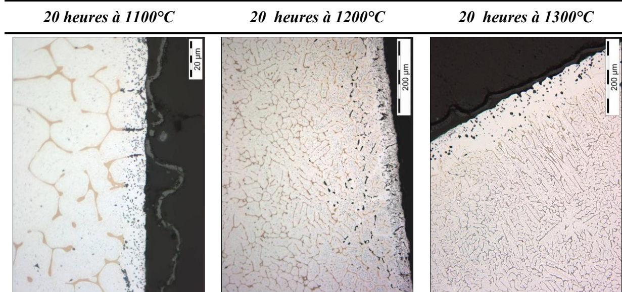
Figure 107 : Micrographies de l'alliage Cr-8%Ni-8%Al (at.%) après 20 heures d'oxydation à l'air à 1100, 1200 et 1300°C
