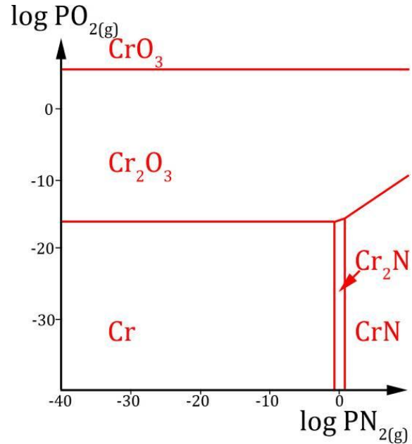
Figure 20 : Diagramme de stabilité thermodynamique des espèces du système Cr-O-N à 1300°C
