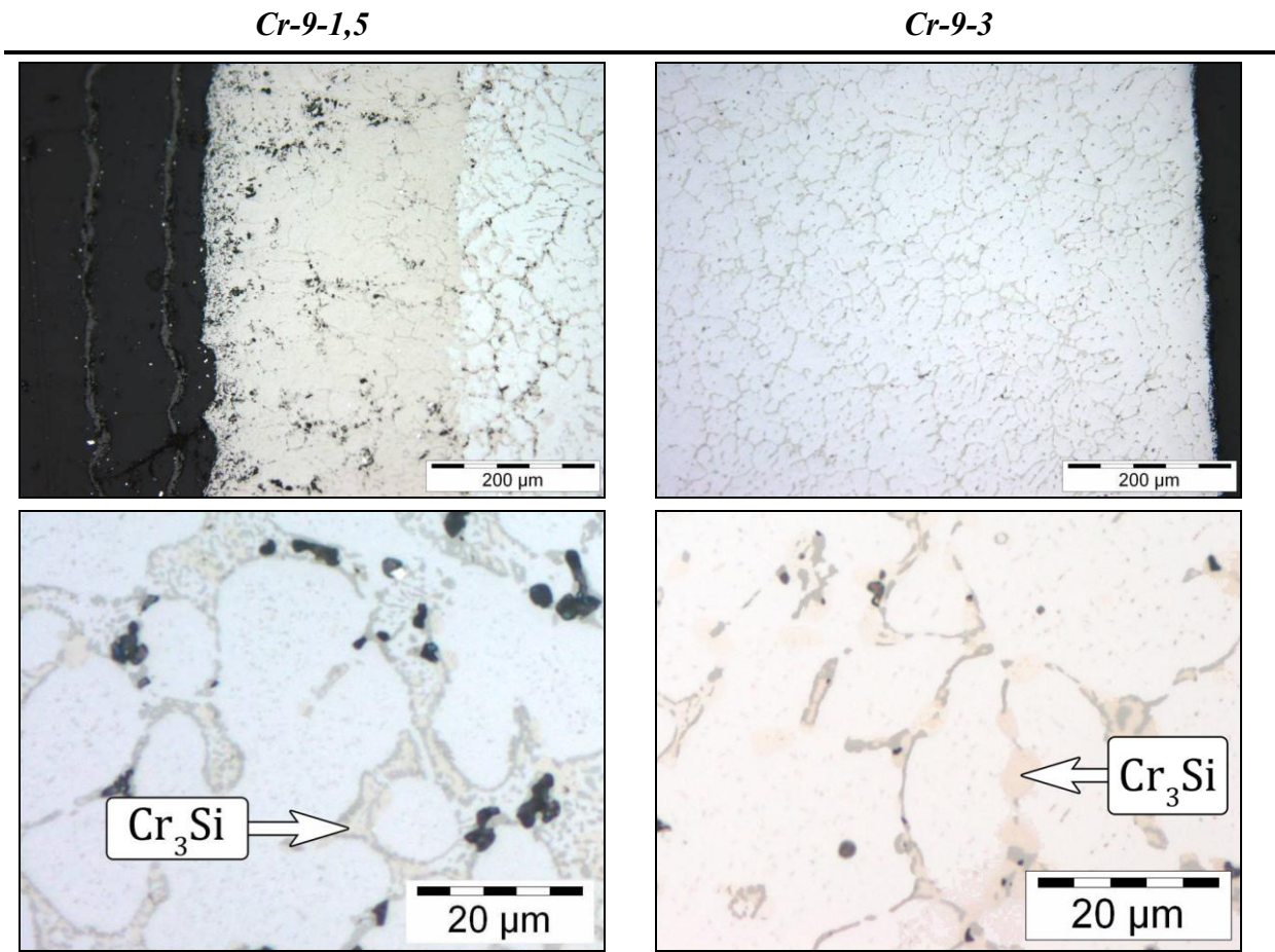
Figure 162 : Faciès d'oxydation des alliages Cr-Ta-Si et transformation des phases de Laves après 15 cycles de 23 heures à 1200°C
