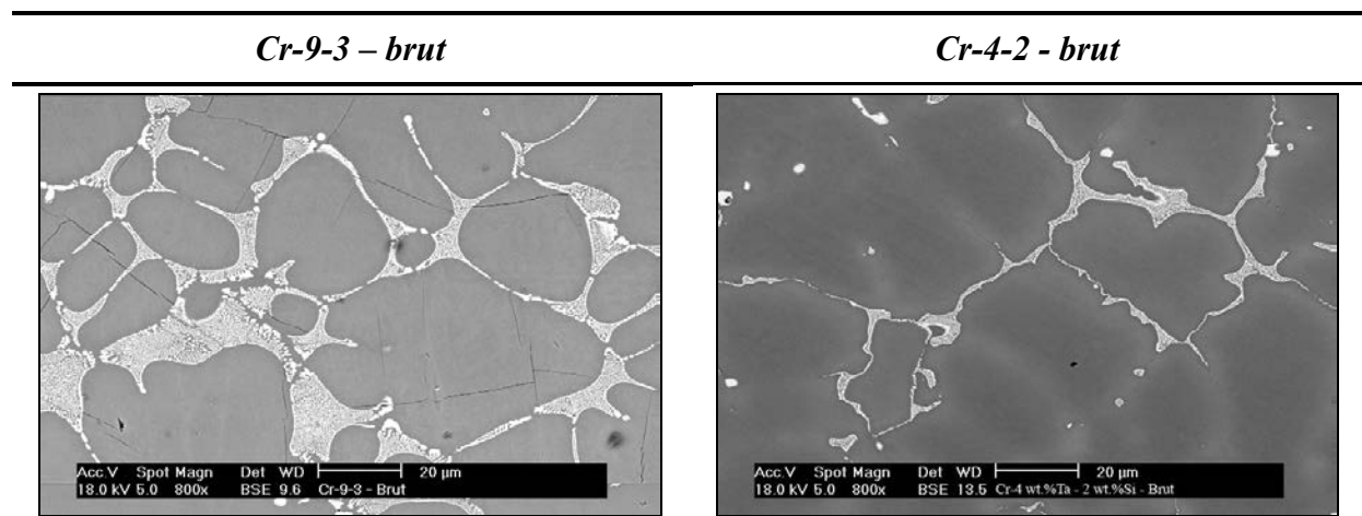
Figure 116 : Microstructures de deux alliages Cr-Ta-Si à l'issue de leur élaboration
