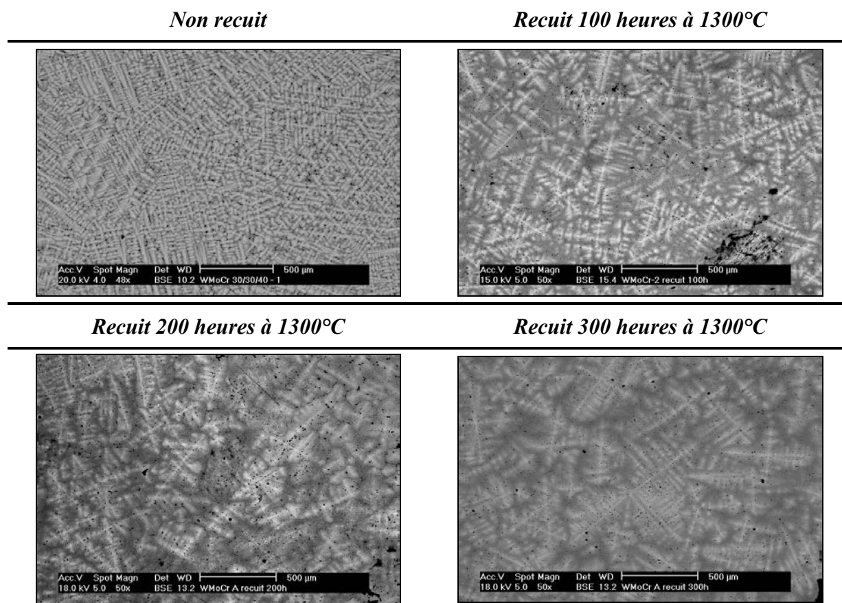
Figure 83 : Images en électrons rétrodiffusés de l'alliage Cr-WMo 1
