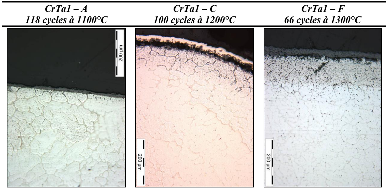
Figure 159 : Micrographies optiques des échantillons CrTa1 après oxydation cycliques entre 1100 et 1300°C
