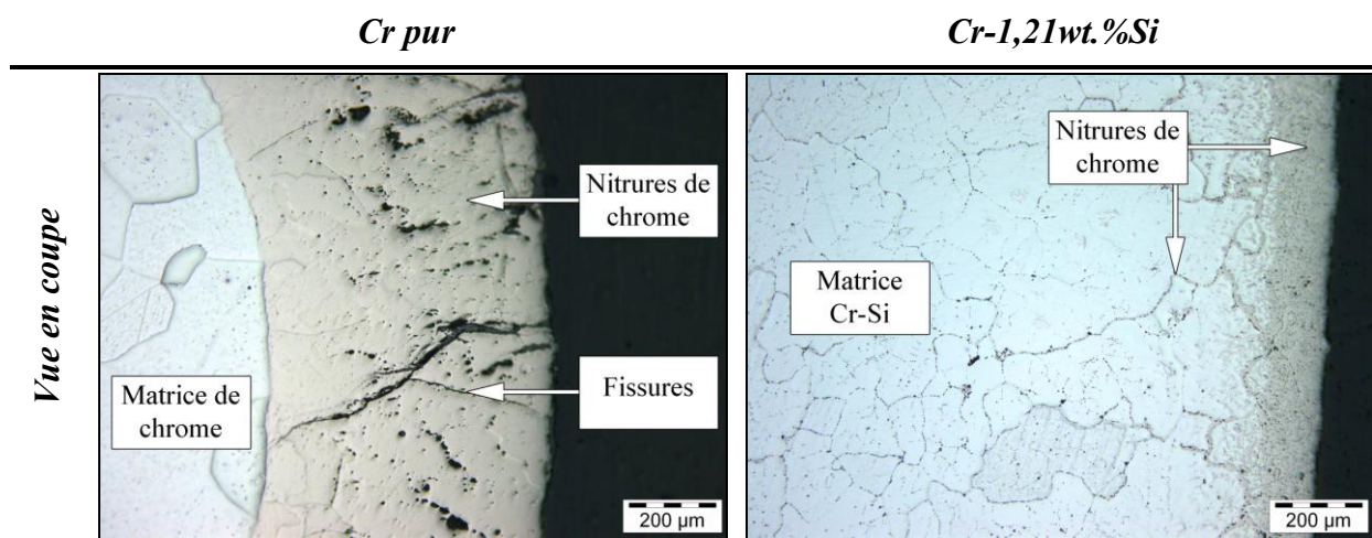
Figure 73 : Micrographies optiques des échantillons Cr et Cr-1,21 wt.%Si après 50 cycles d'une heure à 1300°C.
