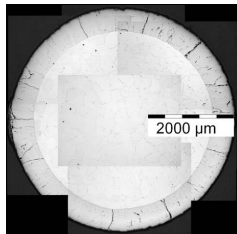
Figure 58 : Faciès de nitruration du chrome HIP 2
