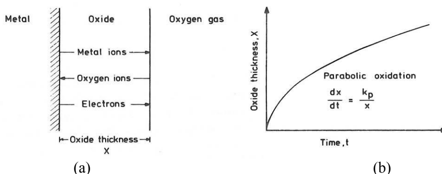
Figure 180 : Représentation schématique des processus de transports au travers d'une couche d'oxyde compacte (a) au cours d'une oxydation haute température de type parabolique (b) [62]
