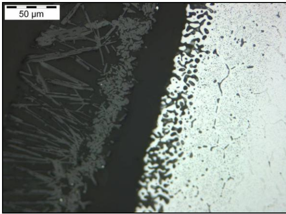
Figure 171 : Faciès de corrosion des alliages Cr-Cr 2 Ta immergés à 1300°C (THA)
