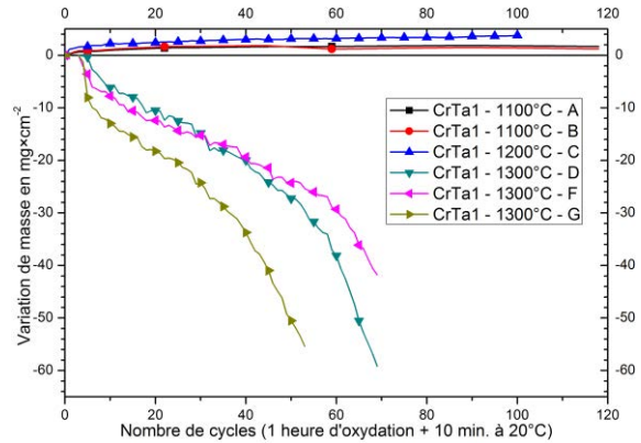
Figure 158 : Résultats d'essais d'oxydation cycliques à 1100°C, 1200°C et 1300°C d'alliages CrTa1
