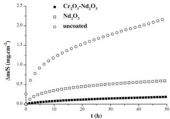
Figure 25 : Amélioration de la tenue en oxydation à 1000°C d'un alliage Fe-30%Cr en présence d'éléments actifs, d'après Chevalier [81]
