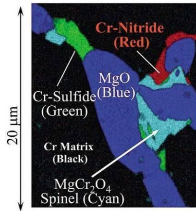
Figure 5 : Cartographie EDS des phases à proximité de particules de MgO/MgCr_2O_4 au sein d'un alliage Cr-6 \text{ wt.}\%MgO , d'après Brady [25]
