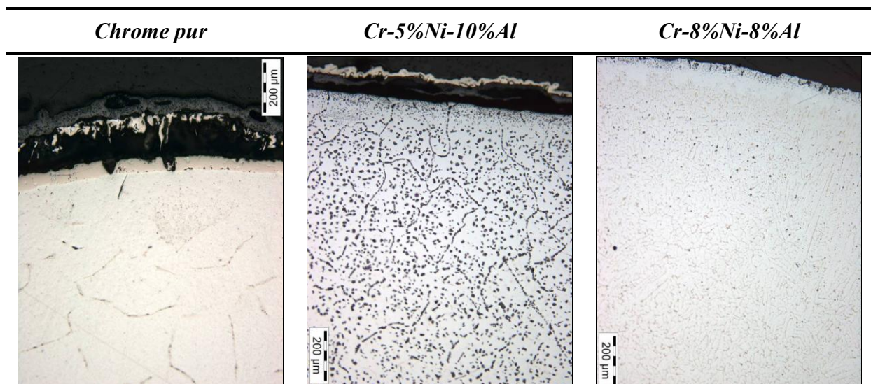
Figure 105 : Micrographies optiques du chrome pur et des alliages Cr-5-10 et Cr-8-8 après oxydation 20 heures à 1300^\circ\text{C}
