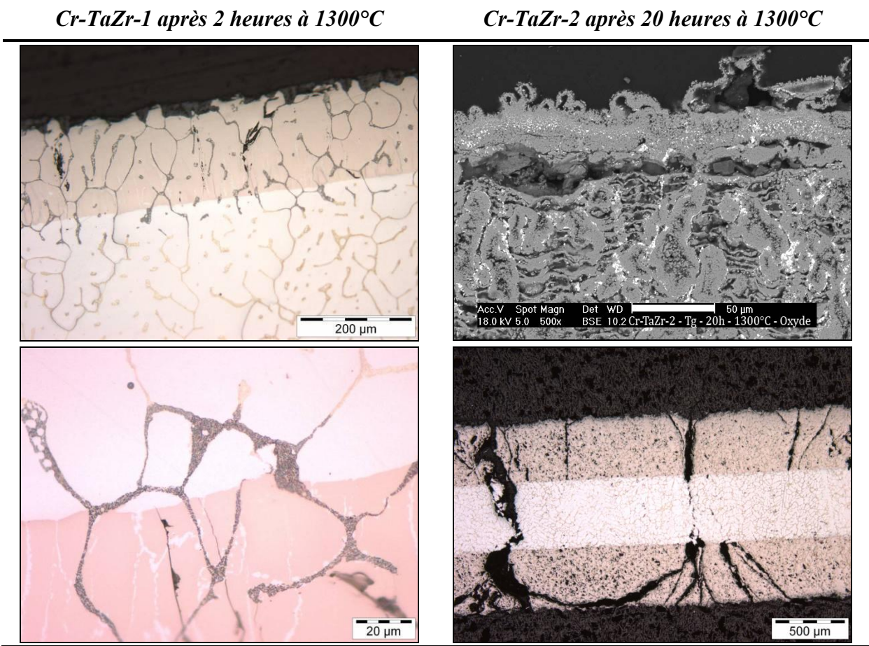
Figure 148 : Micrographies optiques des échantillons Cr-TaZr-1 et Cr-TaZr-2 après oxydation en thermobalance à 1300°C
