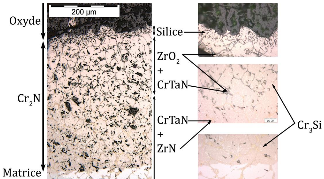
Figure 149 : Répartition des produits d'oxydation au sein de Cr-TaZr-2
