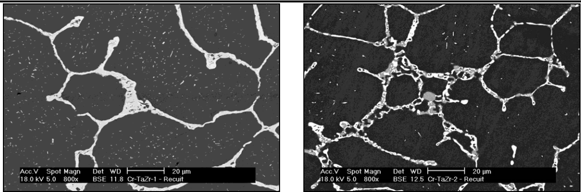
Figure 122 : Micrographies électroniques des alliages Cr-Ta-Zr-(Si) après traitement thermique
