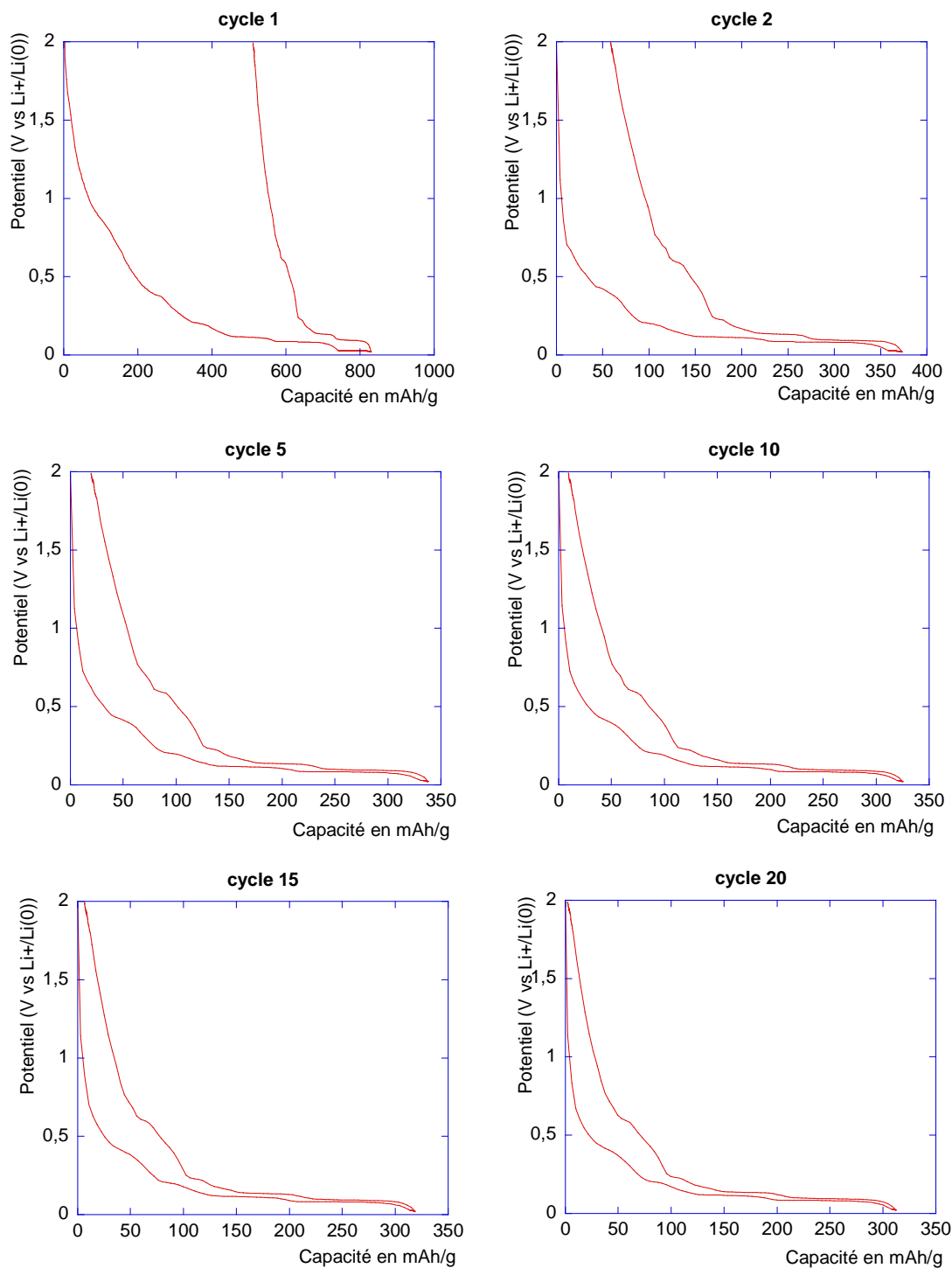
Figure 3.78 : Cycles galvanostatiques de charge/décharge du produit lavé GE12 sous un courant de 10\mu\text{A}/\text{mg}
